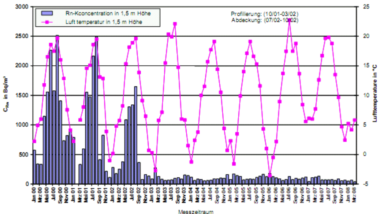
Abb. 2: Entwicklung der Radonkonzentration im Bereich Edelhofweg der Halde 66/207
