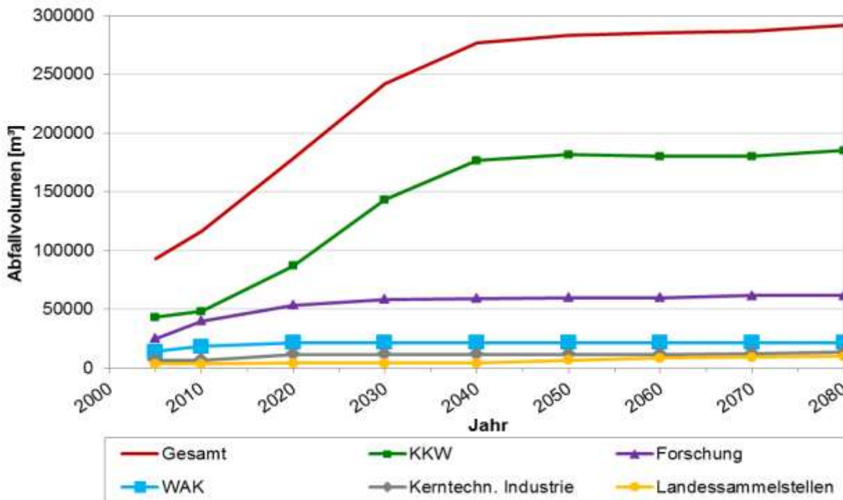
Abbildung D-19: Zeitlicher Verlauf des kumulierten Anfalls radioaktiver Abfälle mit vernachlässigbarer Wärmeentwicklung als Abfallgebinderolumen in m 3 bis zum Jahr 2080
