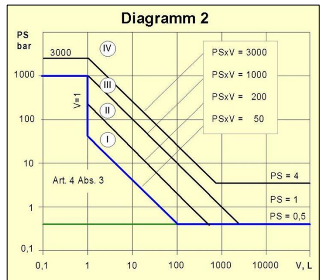
Bild 5: Diagramm 2 nach Anhang II der DGRL für Behälter für Gase (auch überhitzte Flüssigkeiten) der Fluidgruppe 2
