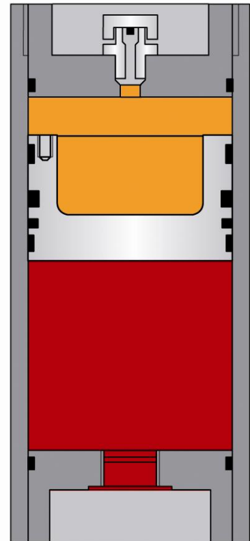
Bild 4: Kolbenspeicher, gefüllt
