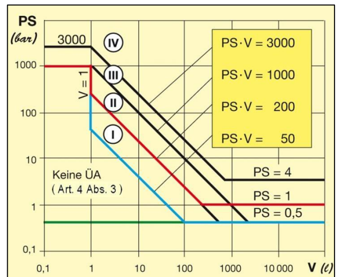
Bild 6: Diagramm 2 nach Anhang II der DGRL für Behälter für Gase (auch überhitzte Flüssigkeiten) der Fluidgruppe 2 mit Prüfstufen für die Prüfung vor Inbetriebnahme (§15 BetrSichV)
