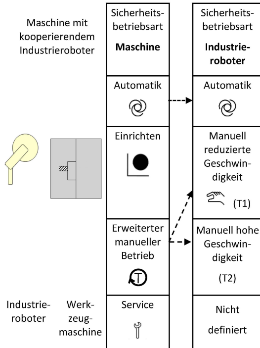
Abbildung 3 – Beispiel einer Verknüpfung von sicherheitsbezogenen Betriebsarten zwischen Werkzeugmaschinen und einem Industrieroboter
