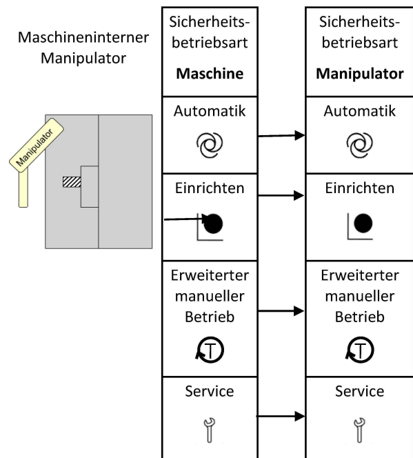
Abbildung 4 – Beispiel einer Verknüpfung von sicherheitsbezogenen Betriebsarten einer Maschine mit sicherheitsbezogenen Betriebsarten eines maschineninternen Manipulators
