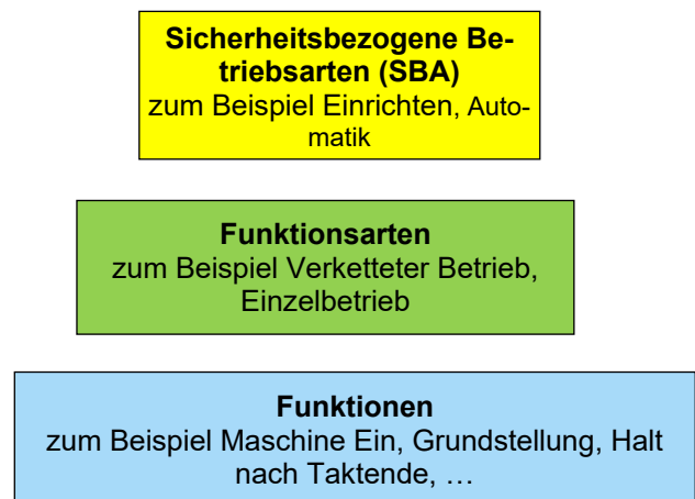
Abbildung 1 – Beispiel für hierarchischen Aufbau unterhalb der sicherheitsbezogenen Betriebsarten
