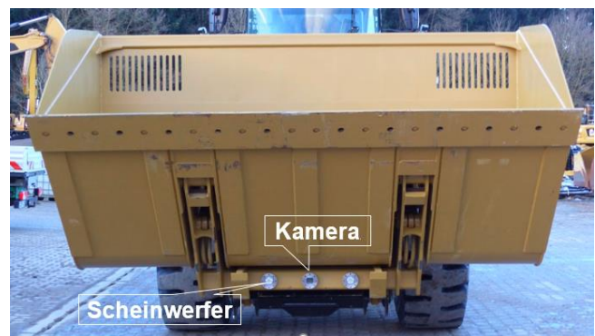
Bild 5: Kamera unterhalb der Ladeschaufel
