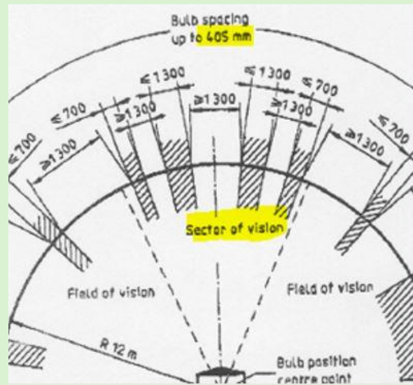
Bild 16: ISO 5006-2:1993, Bild 3, Radlader über 24 t
