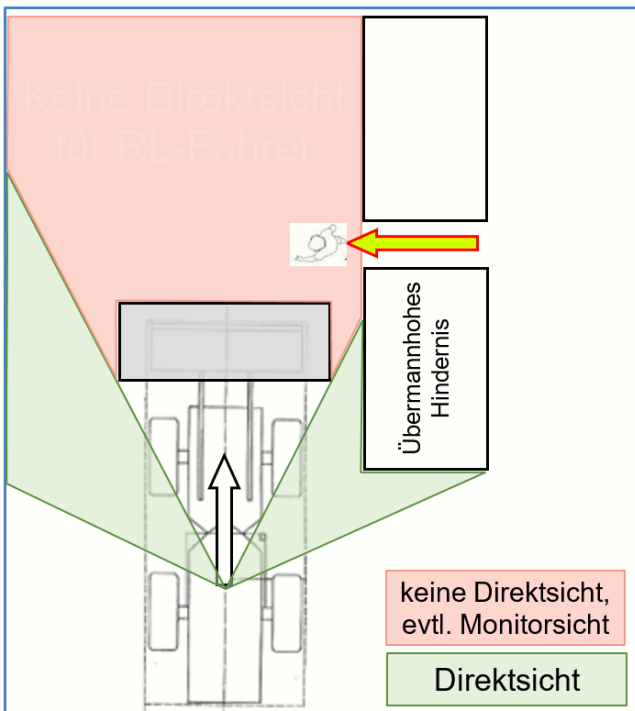
Bild 10: Hindernisse am Fahrbahnrand
