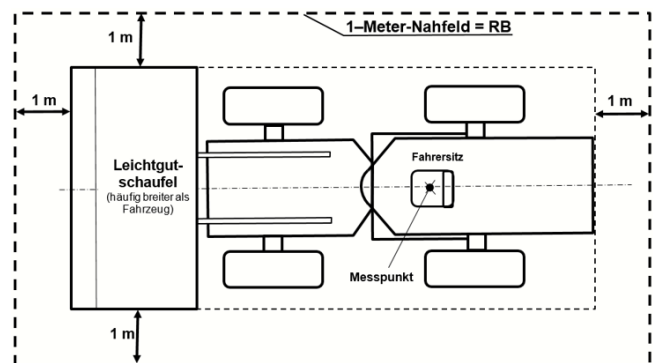
Bild 3: 1-Meter-Nahfeld – Rechteckige Umgebungslinie (RB) im Abstand von 1 Meter von der Maschine für die Nahbereichsmessung mit Prüfkörper
