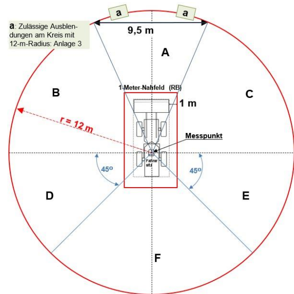
Bild 2: Kreis mit 12-m-Radius und 1-Meter-Nahfeld (siehe Anlage 4)
