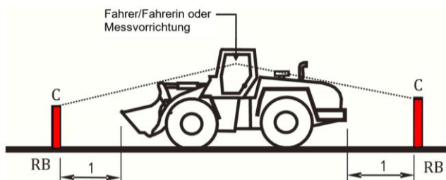
Bild 4: 1-Meter-Nahfeld - Nahbereichsmessung mit 1,2 bis 1,5 Meter hohem Prüfkörper (rot) - siehe Pkt. 4.4
