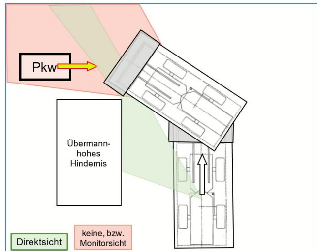
Bild 11: Enges Umfahren von Hindernissen
