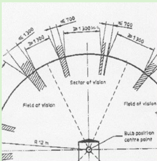
Bild 15: ISO 5006-2:1993, Bild 1, Radlader bis 24 t
