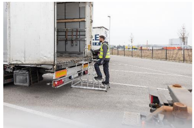
Abbildung 6 – Aufstiegstreppe/Tritt Mobile Treppe mit breiten Stufen, feststellbaren Rollen und Handlauf
