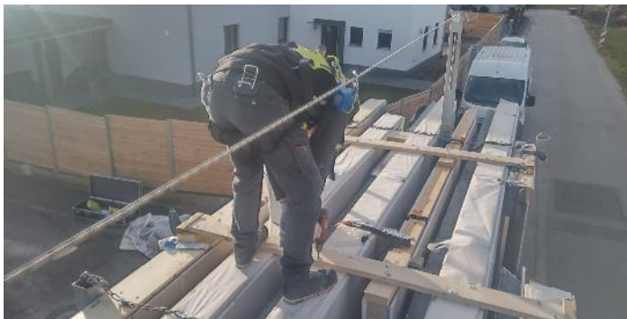
Abbildung 40 – Personensicherung an LifeLine Anschlagpunkt in 1,20 m Höhe an mitlaufendem Auffanggerät
