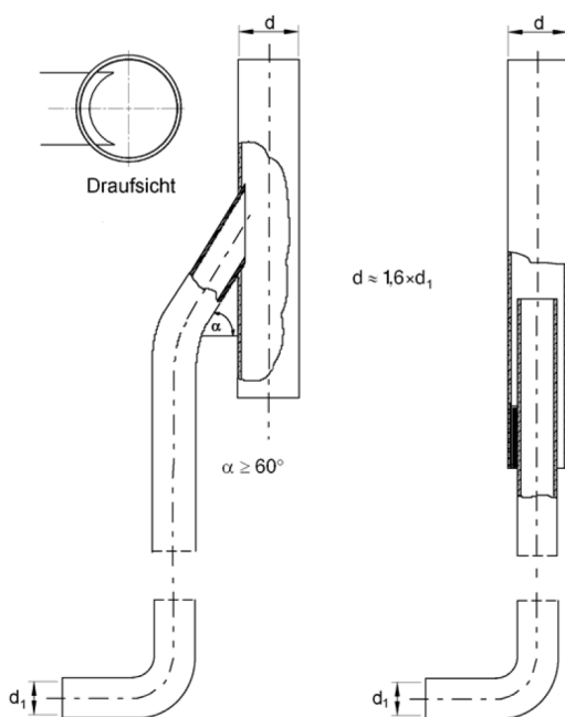
Abbildung 1 Beispiel für eine Ausbläser-Geometrie (aus DVGW G 442 [1])
