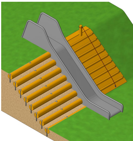
Abb. 8 Beispiel einer Hangrutsche mit seitlichem Freiraum
