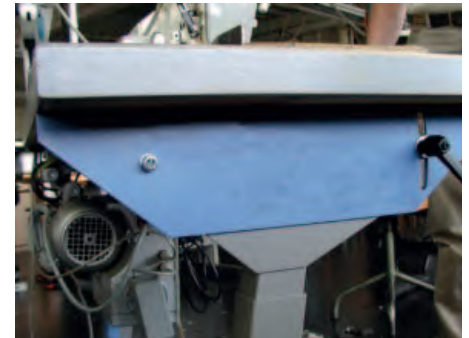
Abb. 27: neue Auflagen für Tischplatte (beidseitig) als Schwenkvorrichtung montiert
