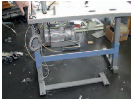
Abb. 26: Traverse ausgewechselt, damit Beinfreiraum in der Breite vergrößert
