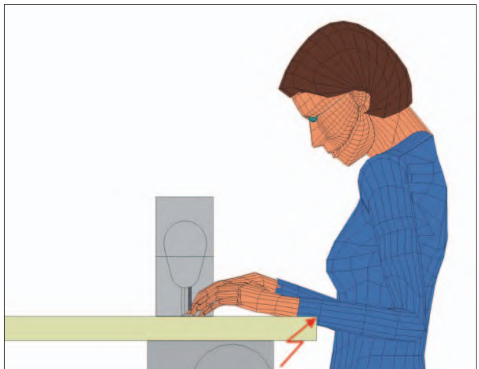
Abb. 12b: Gefahr von Druckstellen an den Unterarmstreckseiten und Einschränkung der Hand-Arm-Bewegungen durch die Tischvorderkante einer Flachbettnähmaschine
