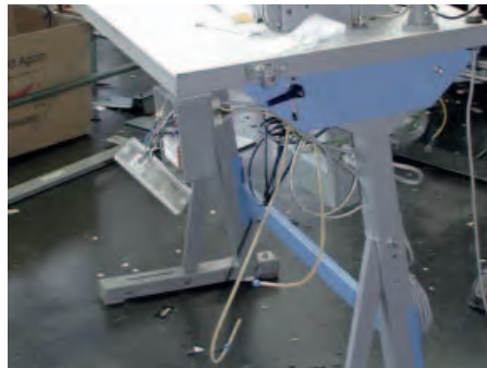
Abb. 28: Tisch manuell stufenlos bis 1000 mm höhenverstellbar und Platte schwenkbar
