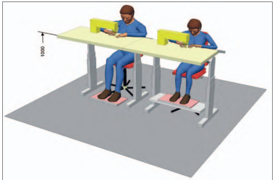
Abb. 3a: Nähmaschinenarbeitsplatz im Sitzen bei fester Tischhöhe (1000 mm) mit großer und kleiner Person, bei letzterer mit höhenverstellbarem Fußschalter
