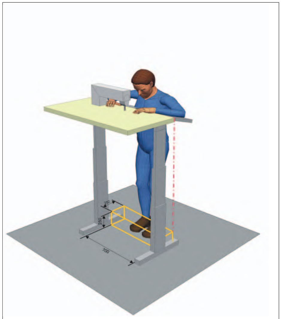
Abb. 8: Mindestmaß für Fußraum beim Stehnäharbeitsplatz
