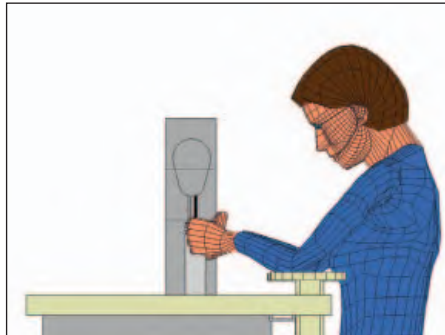
Abb. 15a: Säulennähmaschine mit Armauflagen vorne am Tisch, Schemazeichnung seitlich
