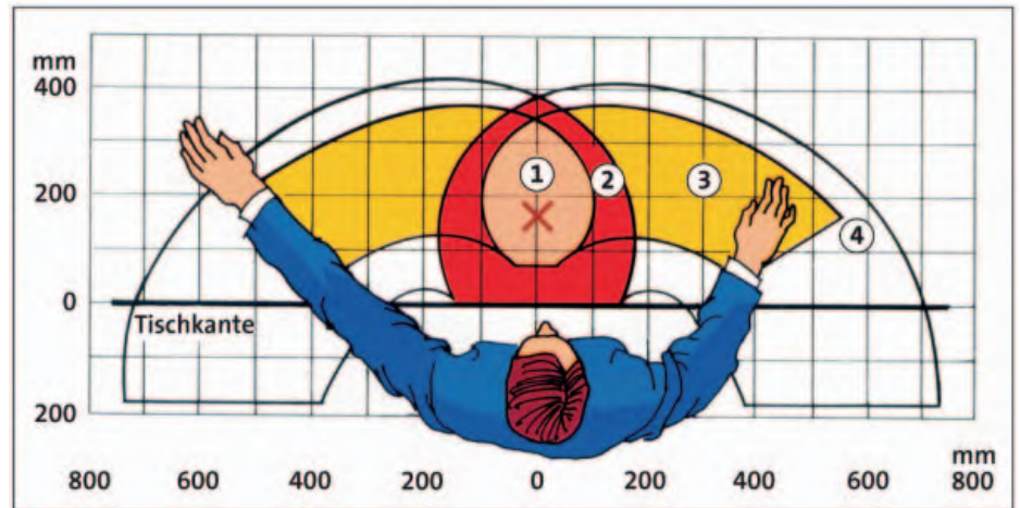
Abb. 20b: Maße des Greifraumes in normaler Arbeitshöhe (aus BGI 523); Nadel (X)
