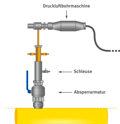
Abb. 29 Schleusenbohrgerät
