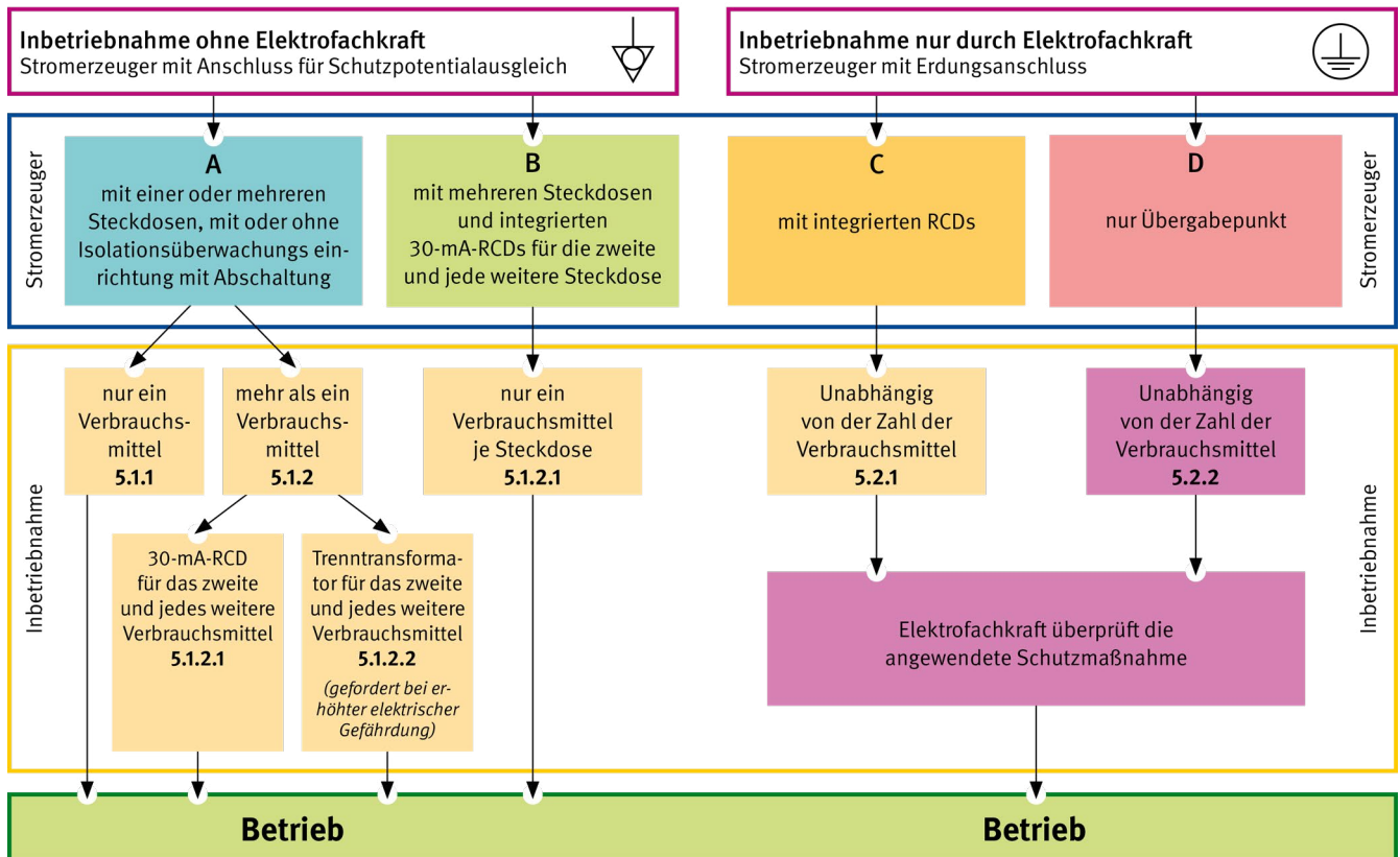
Abb. 14 Schutzpotenzialausgleich/Schutzerdung
