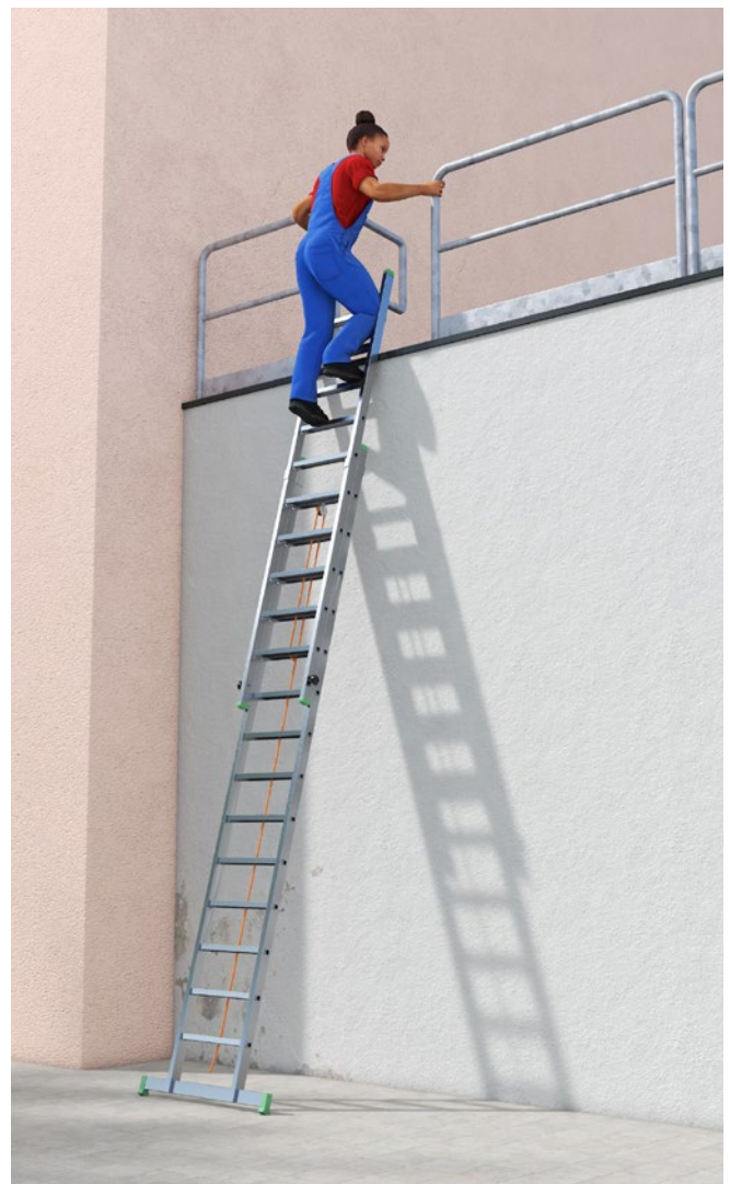
Abb. 18 Schiebeleiter mit Seilzug
