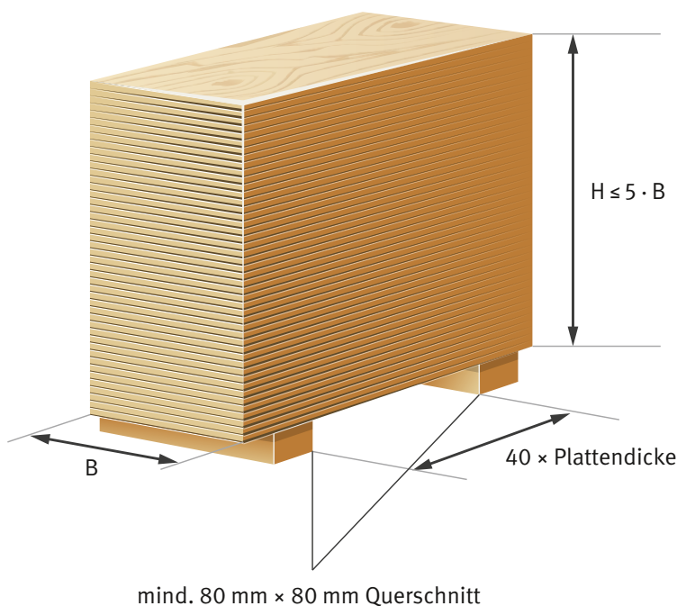
Abb. 56 Plattenstapel
