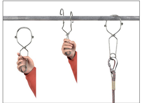
Abb. 6 Anschlagverbindungs-element
