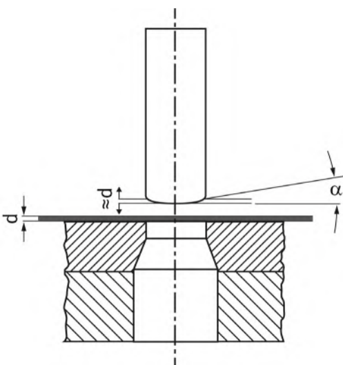
Abb. 28 Schrägschnitte an einem Stanzwerkzeug
