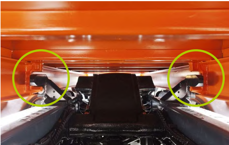
Abb. 39 Abrollbehälter ist über Verriegelungsdorn / Verriegelungsöse formschlüssig gesichert
