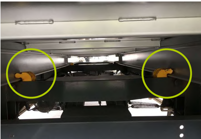
Abb. 40 Pneumatische Klauenverriegelung
