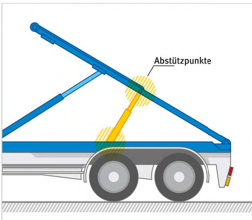
Abb. 21 Abstützpunkte
