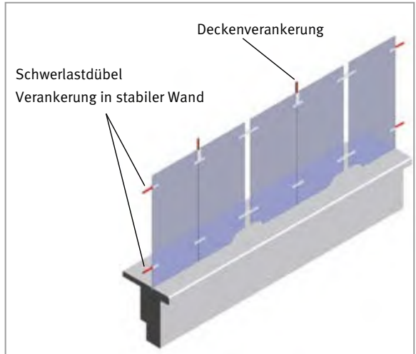
Abb. 23 Durchbruchhemmende Verglasung mit Klammern
