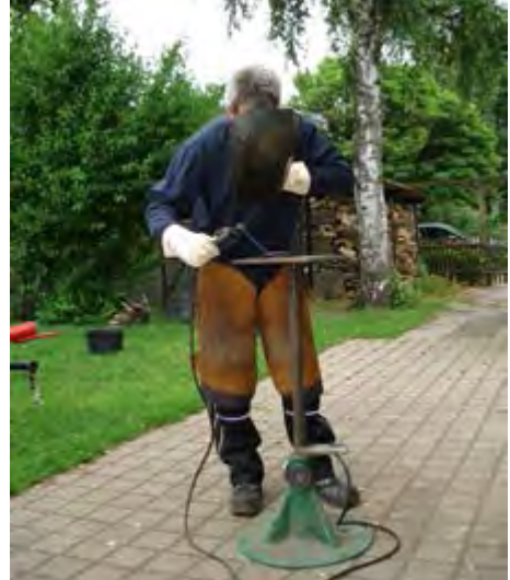
Abb. 5-7 Persönliche Schutzausrüstung beim Schweißen
