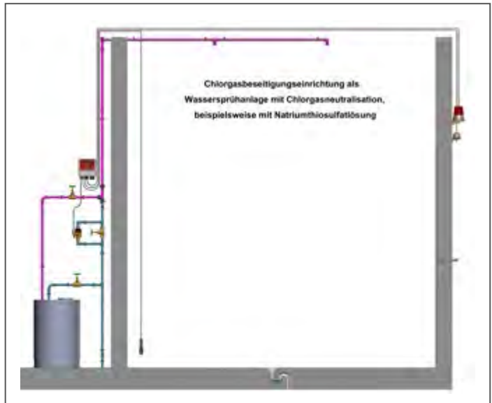
Abb. 4 Natriumthio- sulfatdosierung
