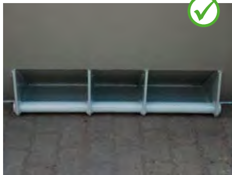
Abb. 16 In das Stirnblech einge- lassene Kipplager
