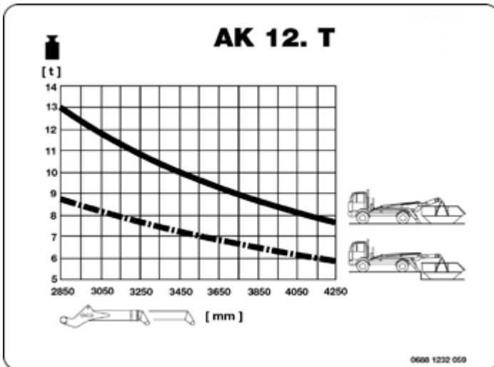
Abb. 6 Hublastdiagramm
