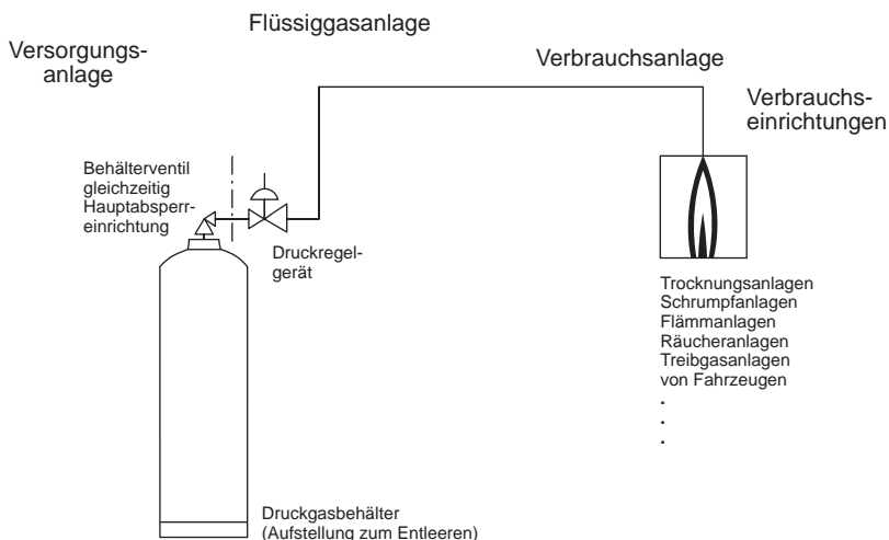
Bild 1: Flüssiggasanlage
