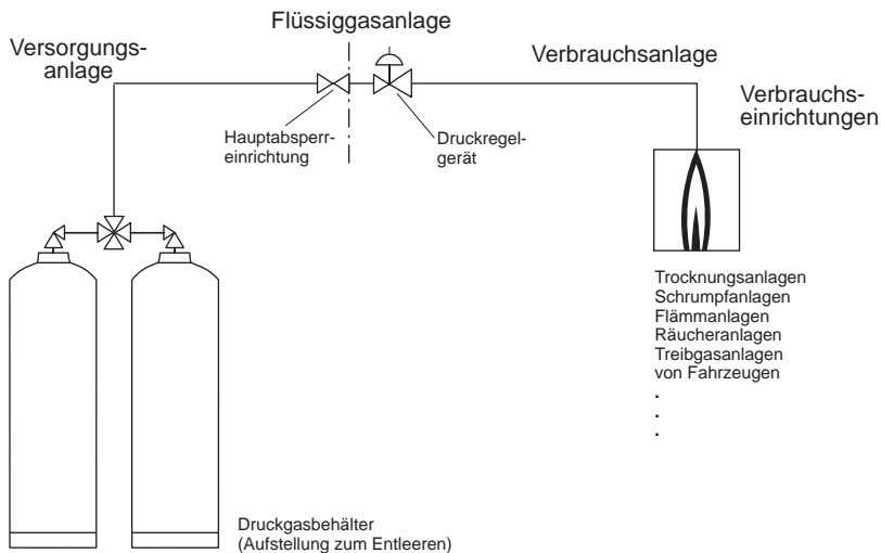
Bild 2: Flüssiggasanlage
