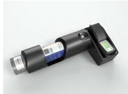
Abb. 30 Vor jedem Einsatz der Messgeräte ist ein Funktionstest nötig.
