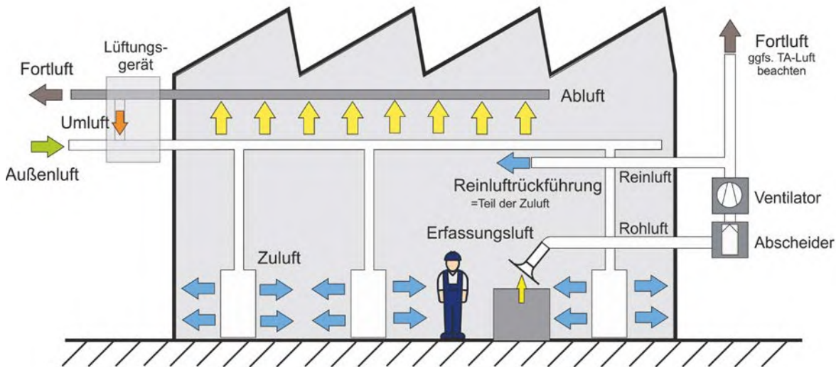
Abb.1 Darstellung der verschiedenen Luftarten
