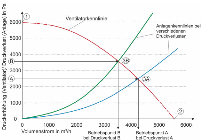
Abb. 11 Grundlagen zu Ventilator- und Anlagenkennlinien
