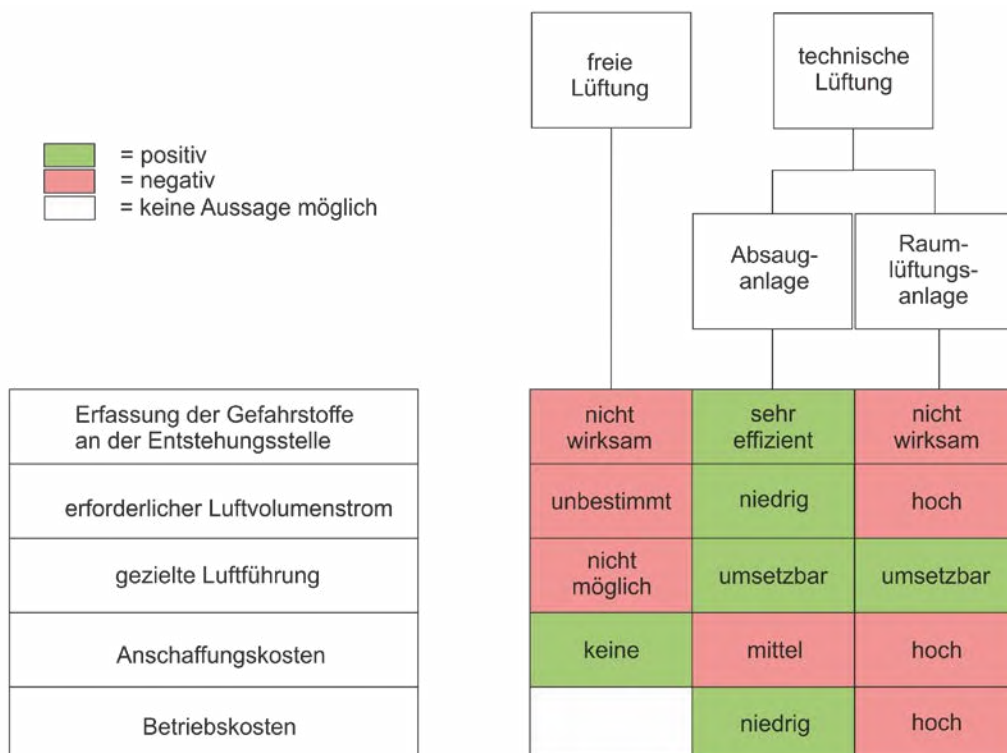
Abb. 2 Beschreibung der Wirksamkeit der Lüftungsarten
