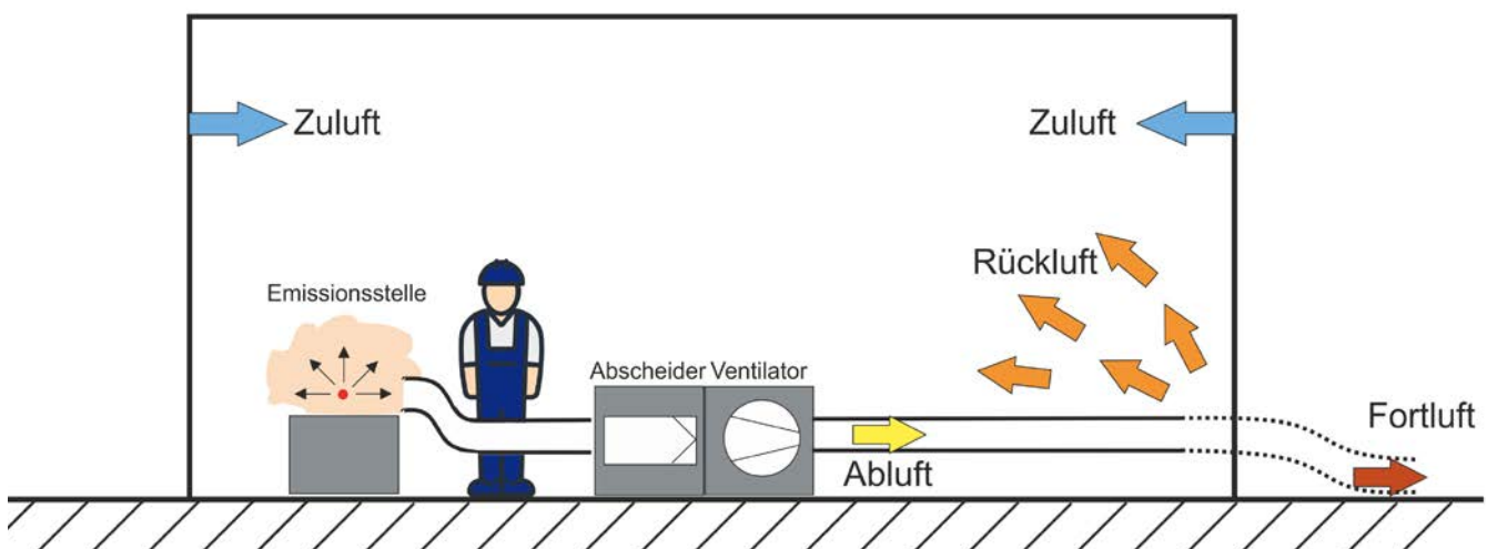
Abb. 12 Luftreiniger auf Baustellen – Absaugung möglichst nahe an der Emissionsstelle
