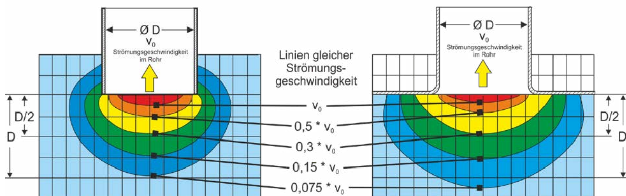
Abb. 3 Vergleich der Saugfelder vor einem Saugrohr und vor einem Saugrohr mit Düsenplatte
