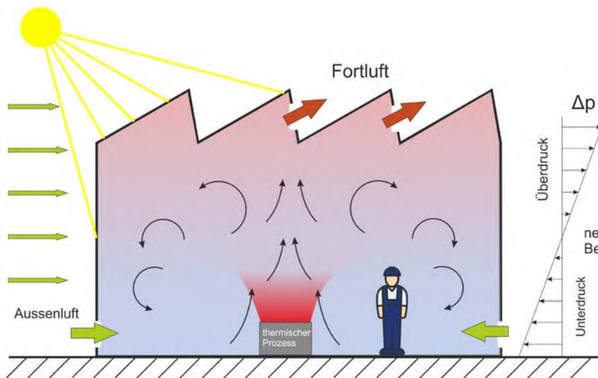
Abb. 7 Prinzip der freien Lüftung mit Darstellung der Druckunterschiede im Innenraum
