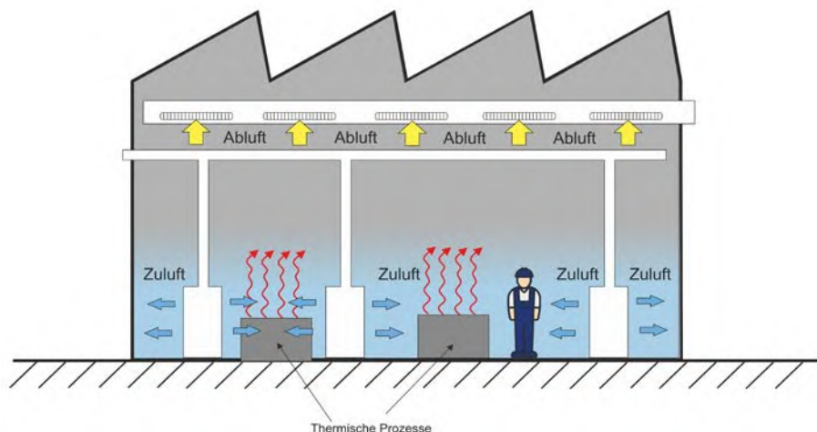
Abb. 5 Prinzip Schichtströmung
