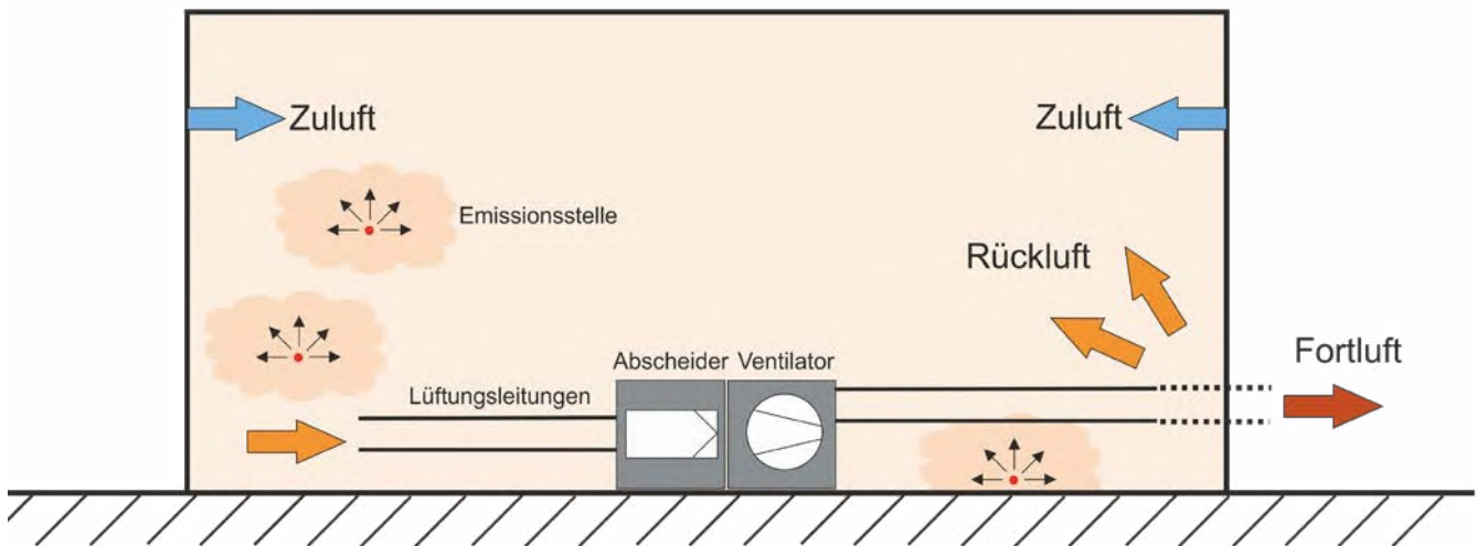
Abb. 13 Luftreiniger auf Baustellen – Reinigung der Raumluft
