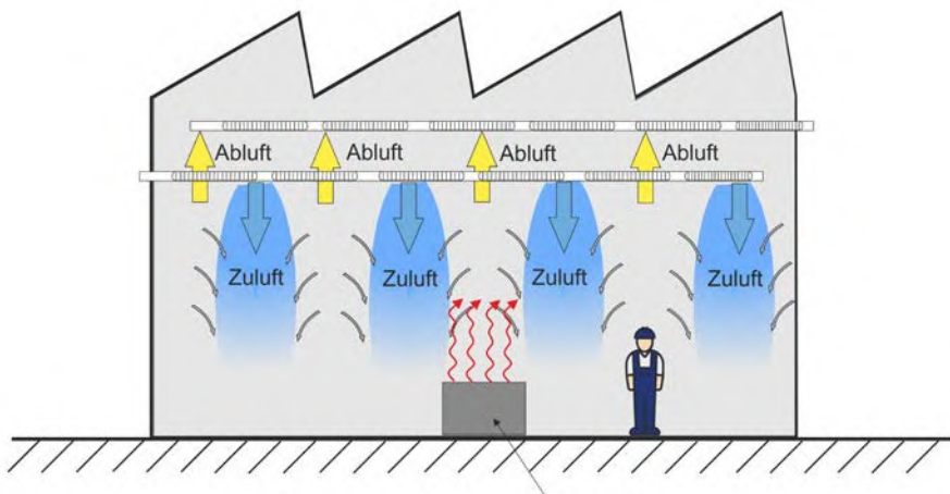
Abb. 6 Prinzip Mischströmung
