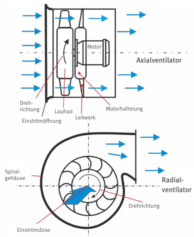
Abb. 10 Bauarten von Ventilatoren
