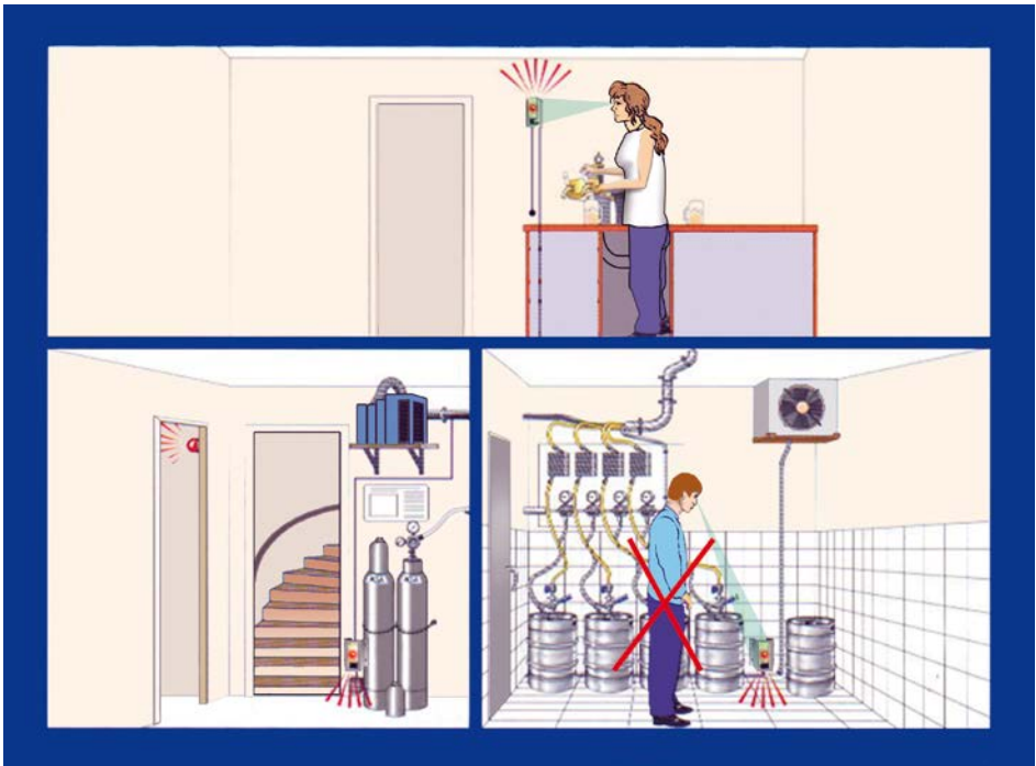
Abb. 13 Beispielhafte Installation der Gaswarnanlage
