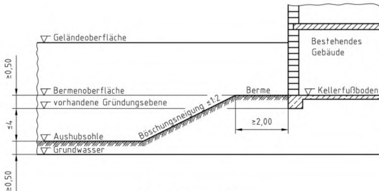
Bild 1 – Bodenaushubgrenzen
