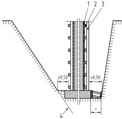
Bild 18 — Arbeitsraum bei geböschten Baugruben (Beispiele)
