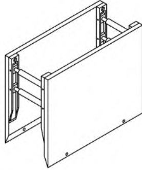
Bild 7 — Beispiel für ein randgestütztes Grabenverbaugerät
