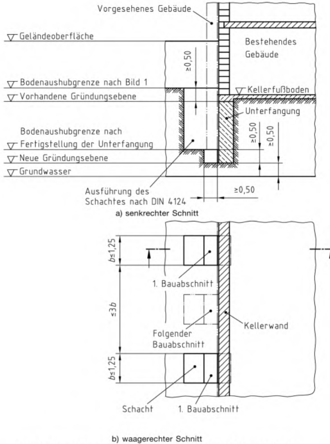
Bild 4 – Unterfangung mit Beispiel für die Abfolge der Bauabschnitte
