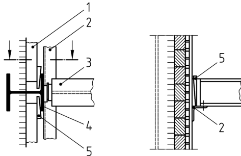
Bild 17 — Einzelheiten einer Trägerbohlwand (Beispiel)
