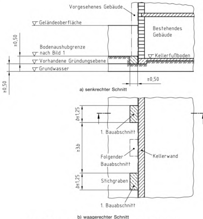
Bild 2 – Gründung mit Beispiel für die Abfolge der Bauabschnitte
