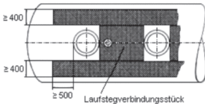
Doppelter Laufsteg mit Verbindungsstück
