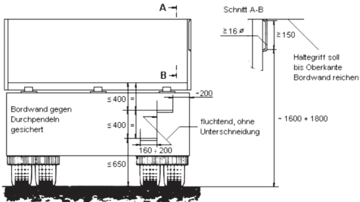
Klappritt-Aufstieg an einer Bordwand
