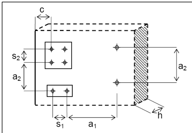
Abbildung 1.2: Dicke des Verankerungsgrundes, Achs- und Randabstände
