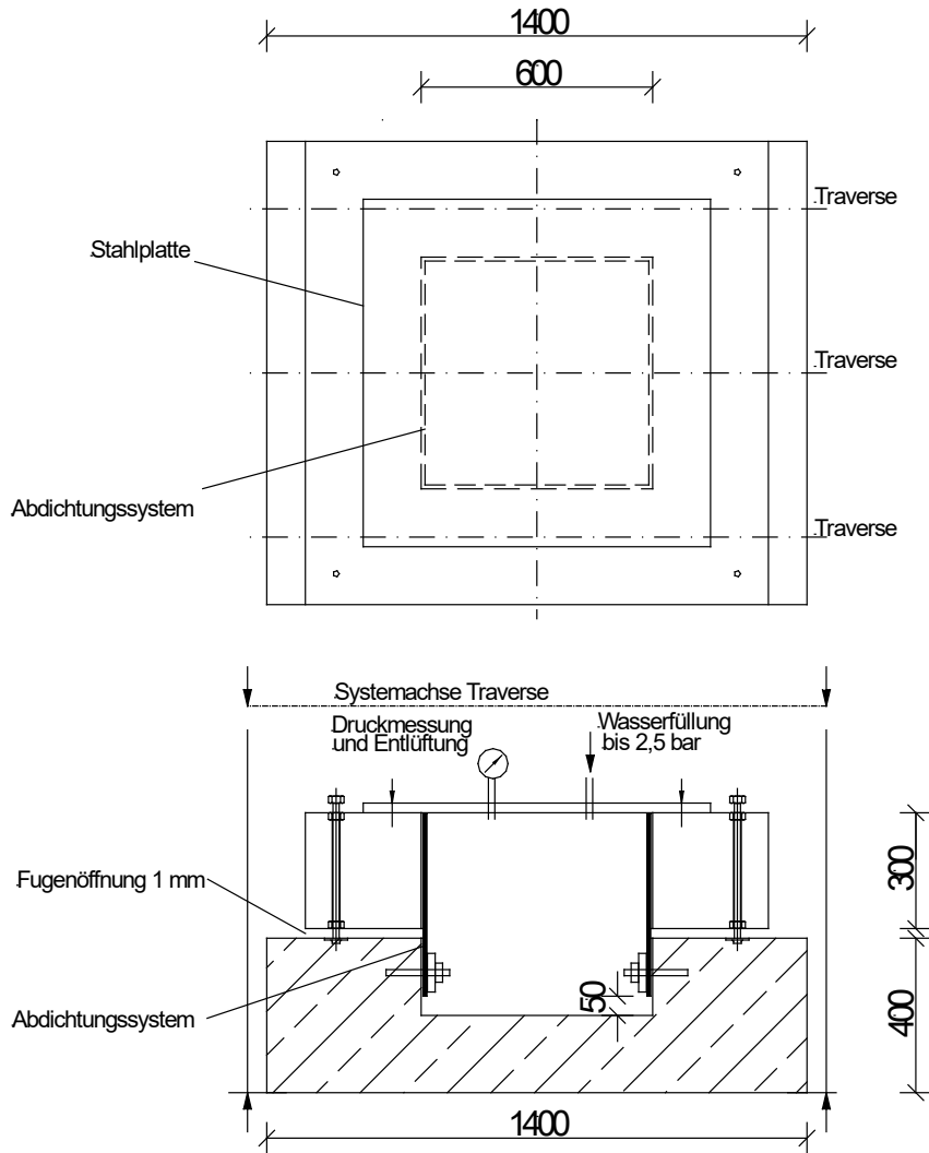
Bild 7: Versuchsaufbau Funktionsprüfung Klemm- und Los-Festflanschkonstruktion, Prinzipskizze
