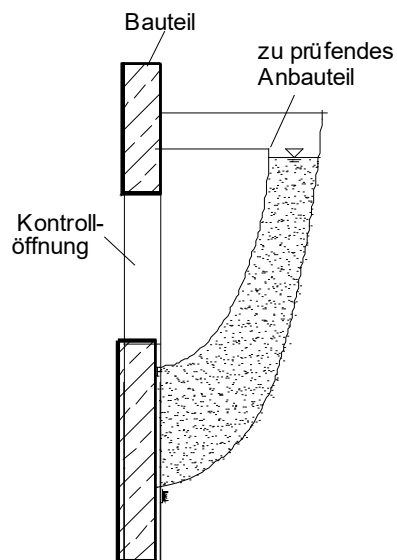
Bild 8: Versuchsaufbau Funktionsprüfung eines Bauteilanschlusses, Prinzipskizze
