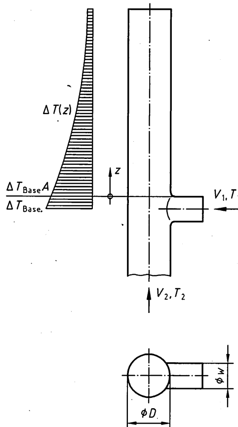
Bild A.1 — Änderung der Temperaturdifferenz \Delta T(z) über die Höhe des Innenrohres
