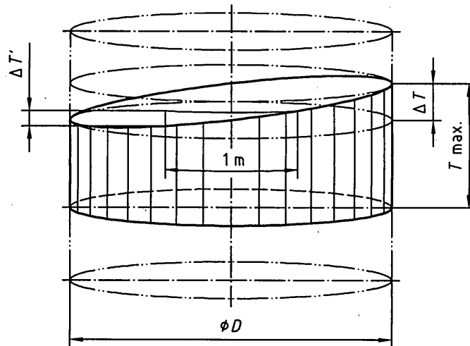
Bild 1 — Lineare Temperaturdifferenz
