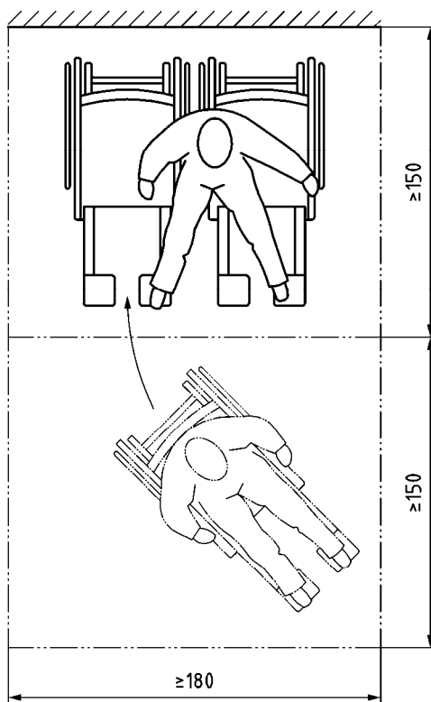
Bild 9 — Platzbedarf für den Rollstuhlabstellplatz einer Person, Bewegungsfläche für Rangieren und Wechsel
