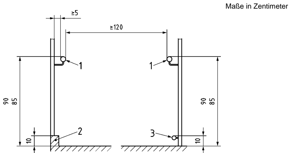
Bild 7 — Rampe, Seitenansicht
