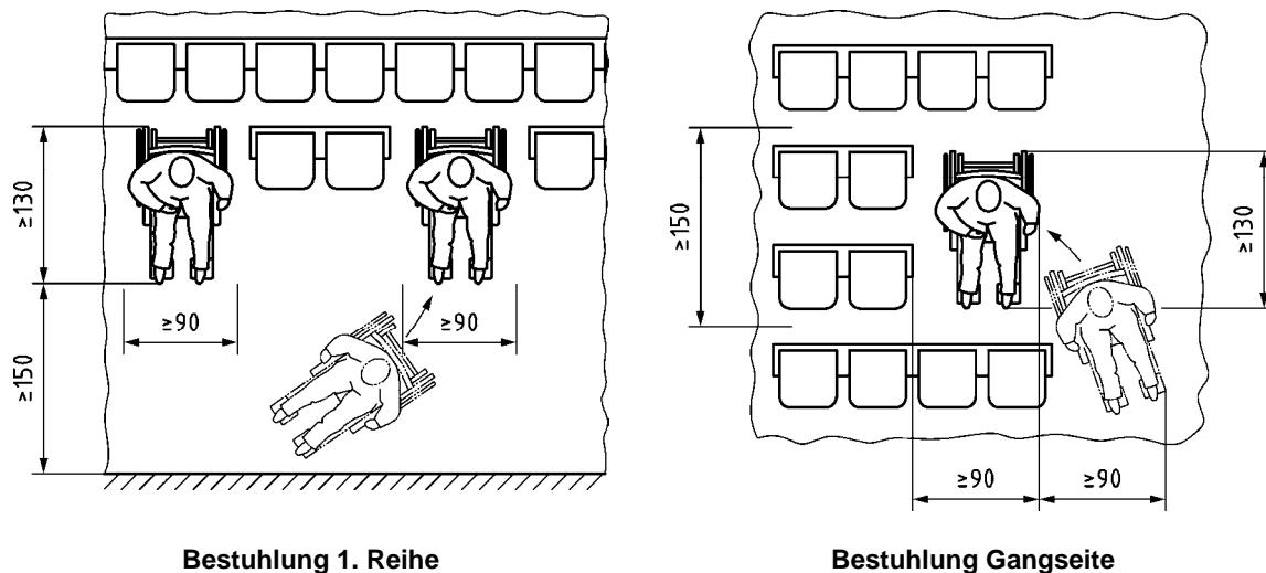
Bild 11 — Beispiele für Rollstuhlplätze in Räumen für Veranstaltungen
