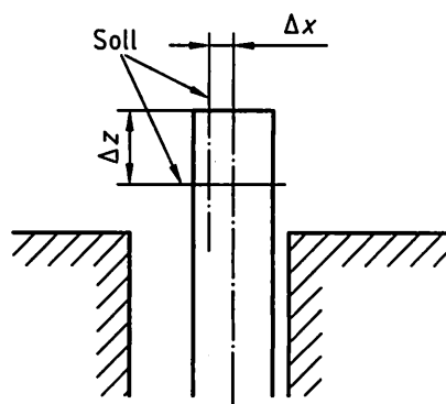
Bild 1 — Zulässige Abweichungen für Ankerbolzen mit Reguliermöglichkeit
