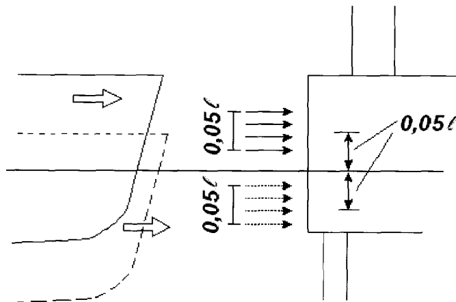
Bild 4.4 — Angaben zu Stoßflächen für Schiffsanprall
