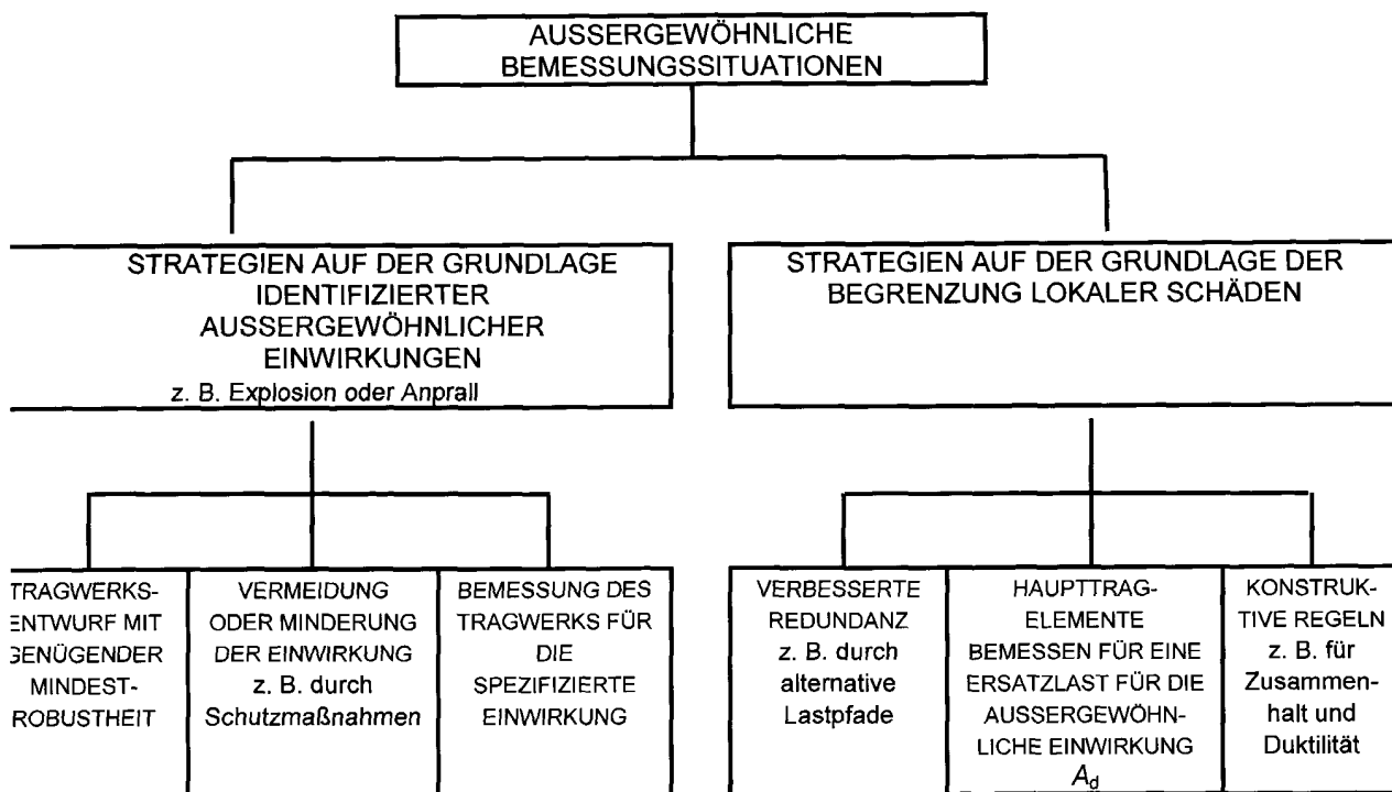
Bild 3.1 — Strategien zur Behandlung außergewöhnlicher Bemessungssituationen
