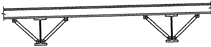
Bild 6.5 — Beispiel für eine Verdrehungsbehinderung
