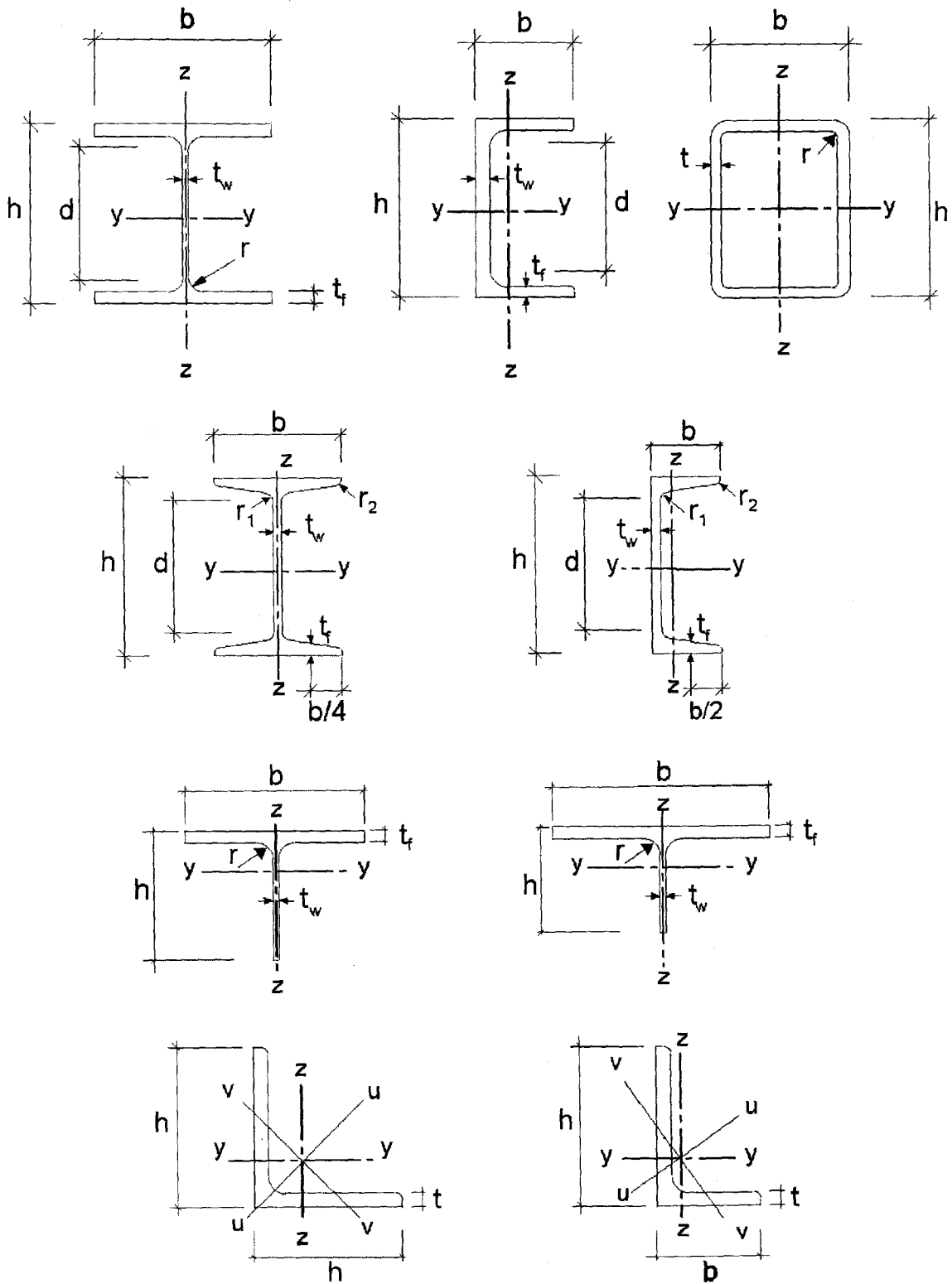
Bild 1.1 — Abmessungen und Achsen von Profilquerschnitten
