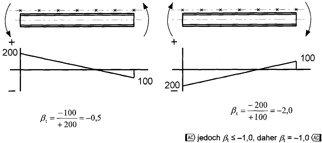
Bild BB.4 — Bestimmung von \beta_t
