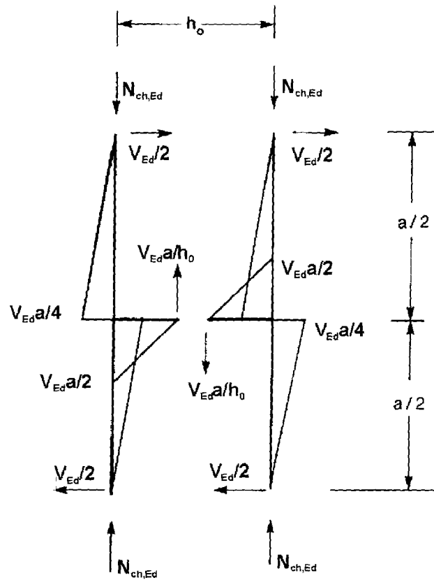
Bild 6.11 — Stabkräfte im Endfeld von Stützen mit Bindeblechen
