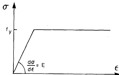
Bild 5.8 — Bi-lineare Spannungs-Dehnungsbeziehung
