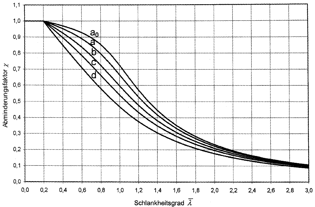
Bild 6.4 — Knicklinien
