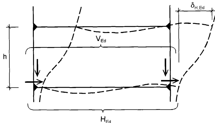
Bild 5.1 — Bezeichnungen zu 5.2.1(4)
