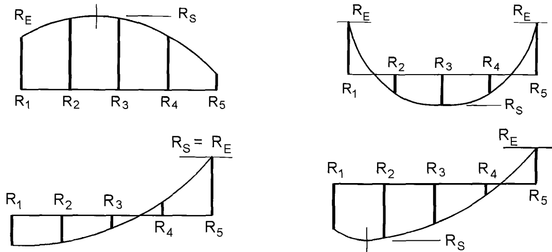
Bild BB.5 — AC Momentenwerte AC
