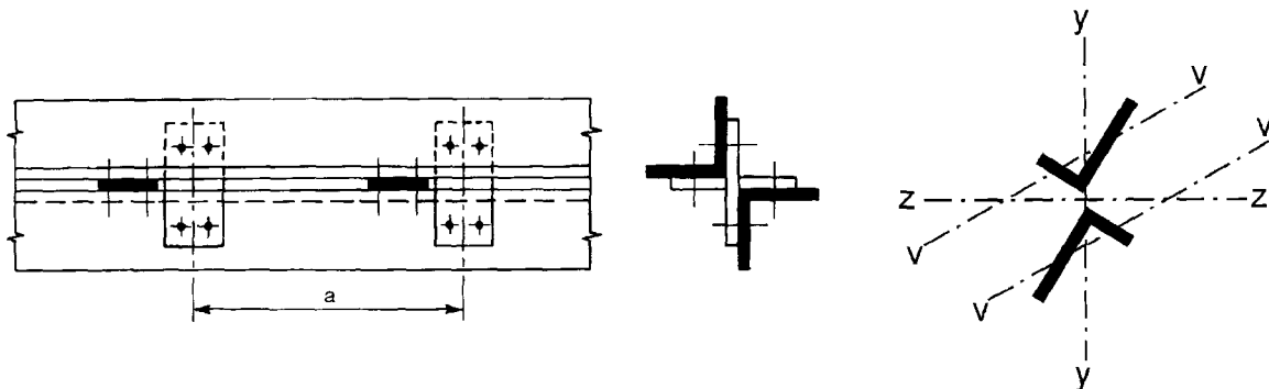
Bild 6.13 — Mehrteilige Bauteile aus über Eck gestellten Winkeln
