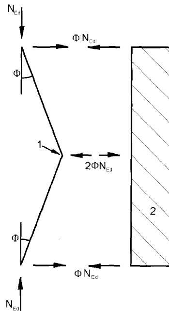
Bild 5.6 — Äquivalente stabilisierende Ersatzkräfte
