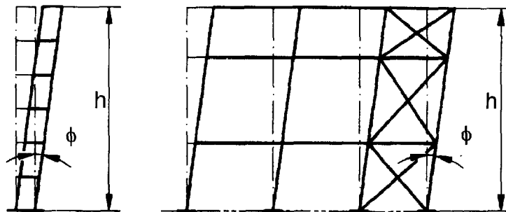
Bild 5.2 — Äquivalente Stützenschiefstellung
