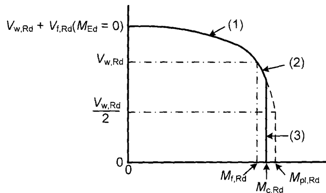
Bild 6.32 — Interaktion von Querkraft- und Biegemomentenbeanspruchbarkeit
