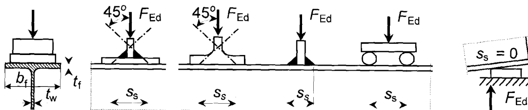
Bild 6.31 — Lasteinleitungslänge
