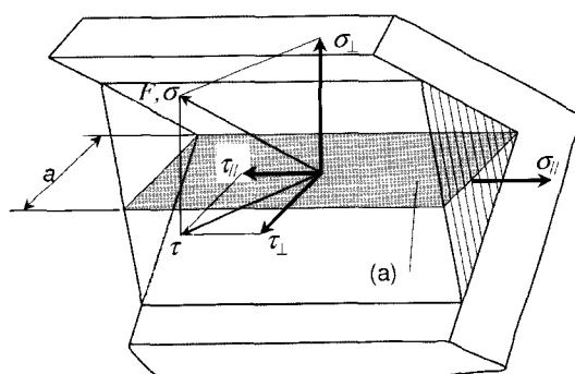
(a) Nahtquerschnitt
