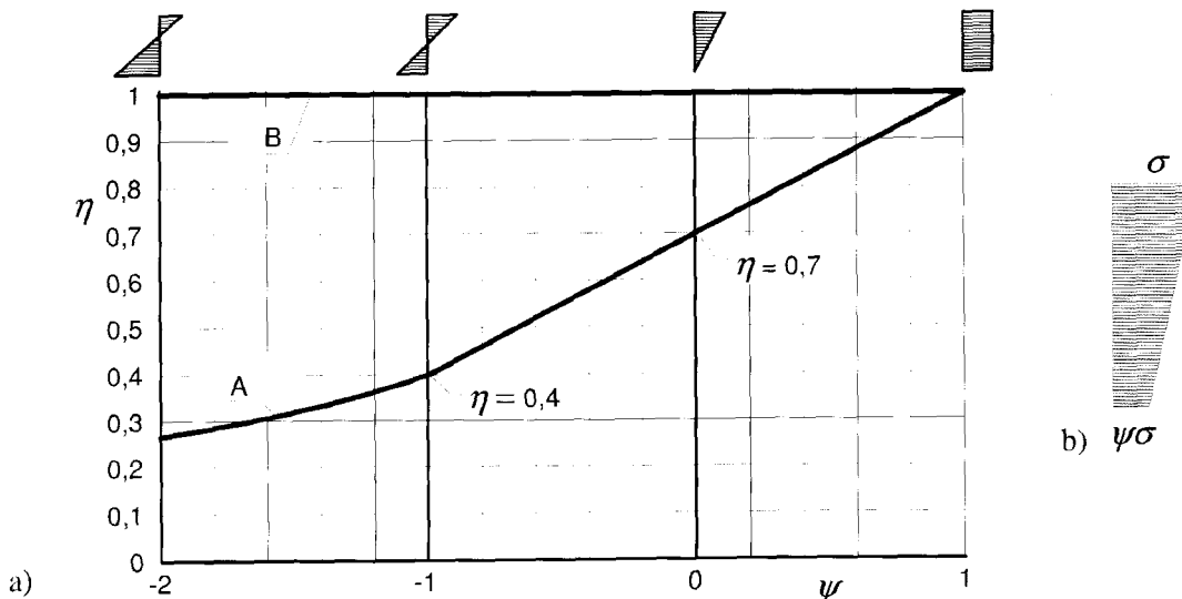
Bild 6.2 —Werte von \eta für ebene innere, beidseitig gehaltene Querschnittsteile mit linearer Spannungsverteilung. Für ebene innere, beidseitig gehaltene Querschnittsteile und für ebene auskragende Querschnittsteile mit größter Druckbeanspruchung am äußeren Rand gilt Linie A. Für ebene auskragende Querschnittsteile mit größter Druckbeanspruchung am inneren Rand gilt Linie B.
