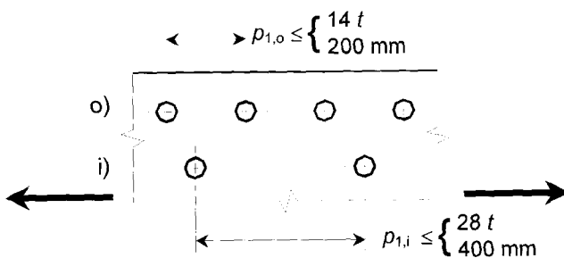
Bild 8.1 — Bezeichnungen der Abstände
