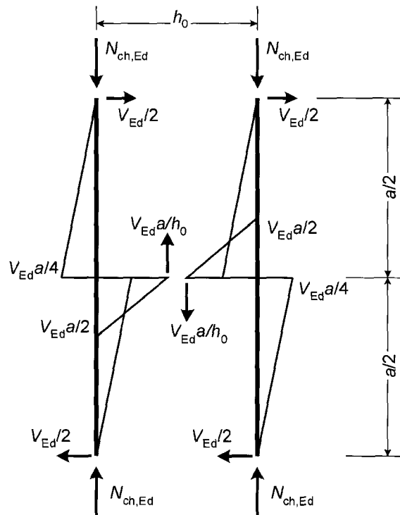
Bild 6.19 — Stabkräfte im Endfeld von Stützen mit Bindeblechen
