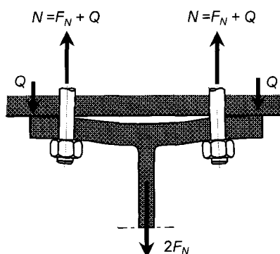
Bild 8.8 — Abstützkräfte (Q)
