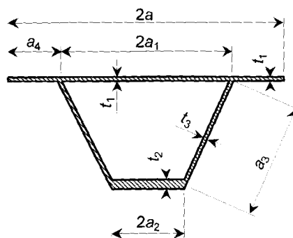
Bild 6.24 — Bezeichnungen beim Querschnitt einer geschlossenen Steife
