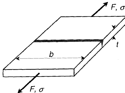
Bild 8.14 — Stumpfnahtheit mit Normalspannungen
