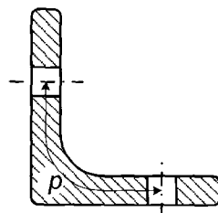
Bild 6.8 — Winkel mit Löchern in beiden Schenkeln
