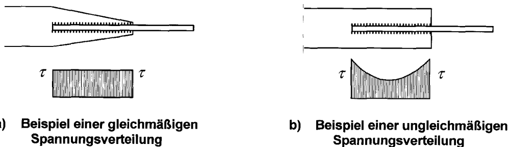
Bild 8.16 — Spannungsverteilungen in Verbindungen mit Kehlnähten \square
