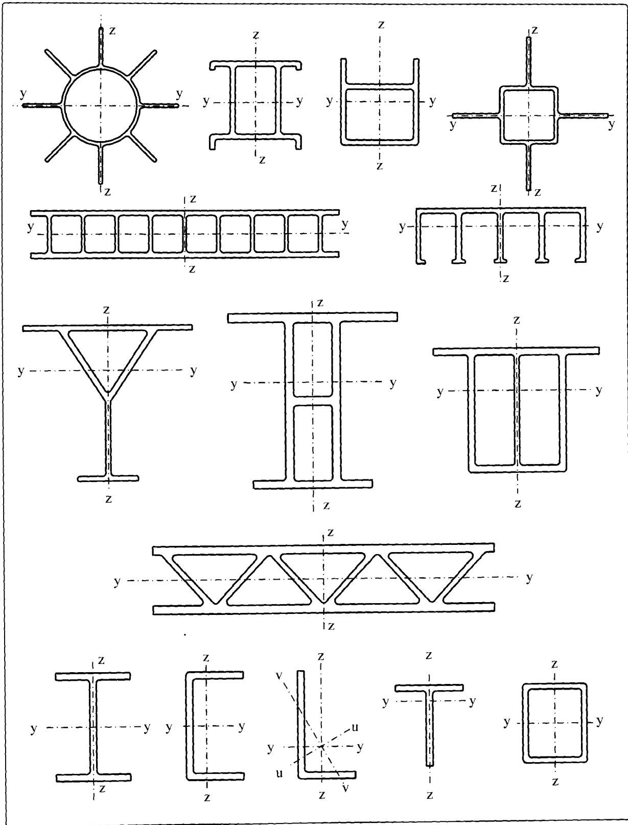
Bild 1.1 — Definition der Achsen für verschiedene Querschnitt
