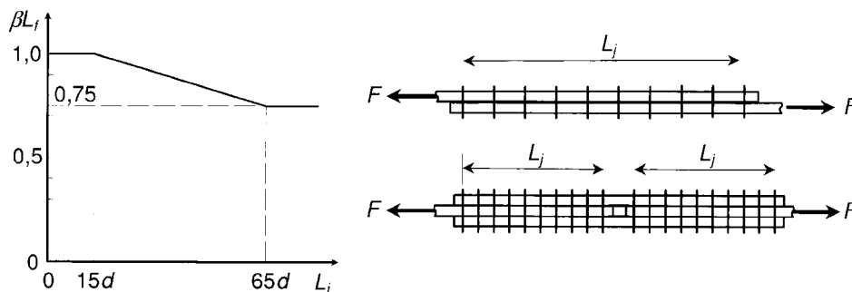
Bild 8.10 — Lange Anschlüsse
