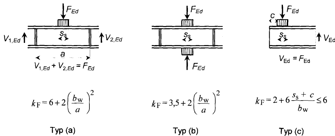
Bild 6.30 — Einleitung von Querlasten und zugehörige Beulwerte
