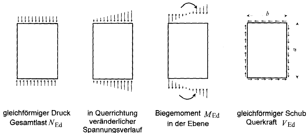
Bild 6.22 — Unausgesteifte Platten
