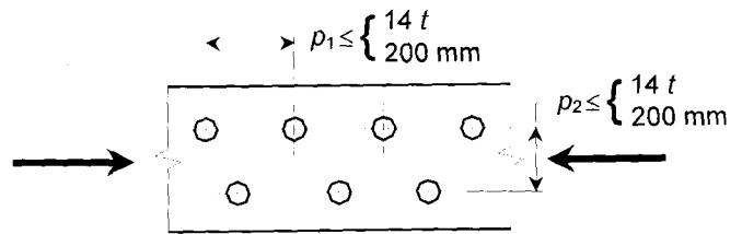
Bild 8.2 — Versetzte Lochanordnung bei druckbeanspruchten Bauteilen
