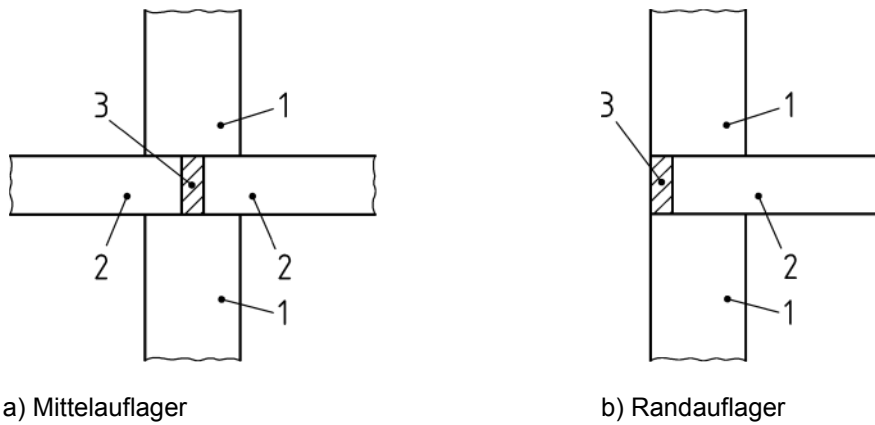
Bild 10.1DE — Beispiel zur Bewehrung einer Wand über der Verbindung zweier Deckenplatten
