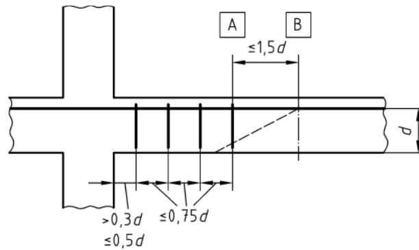
a) Bügelabstände bei Flachdecken
