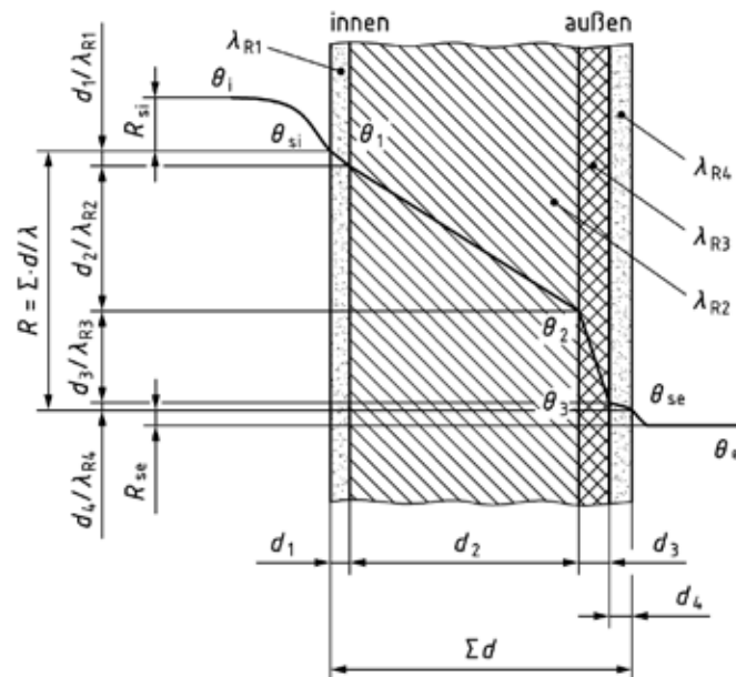
Bild C.1 — Temperaturverteilung über den Querschnitt eines mehrschichtigen Bauteils
