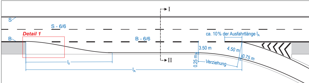
Längen für Ausfädelungstreifen und Verziehung
