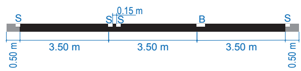
Querschnitt I – II (für Q 2)
