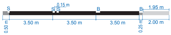
Querschnitt I – II (für Q 3)
