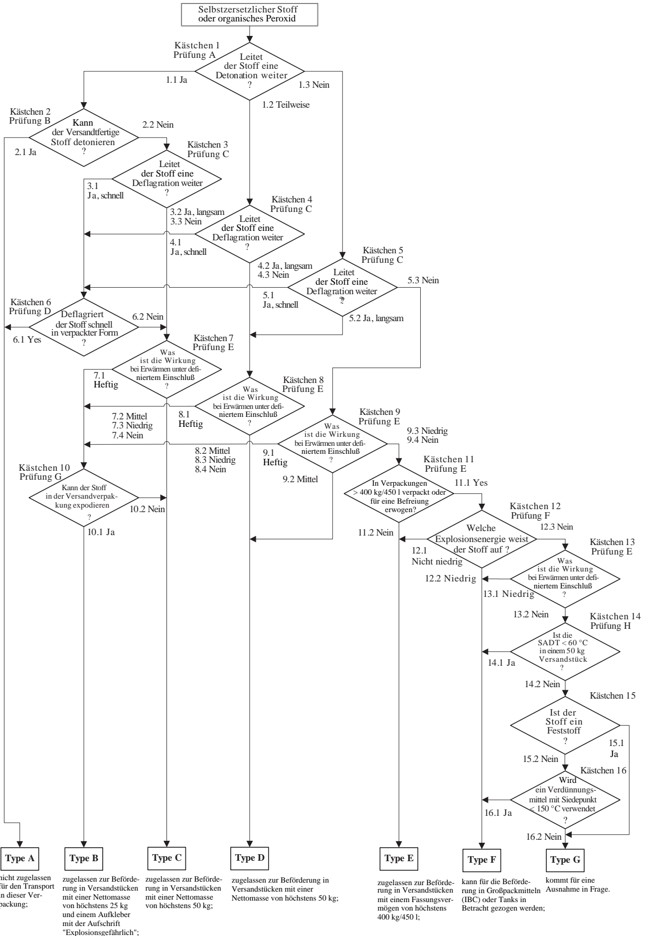
Abbildung 20.1: Flussdiagramm für selbstzersetzliche Stoffe und organische Peroxide
