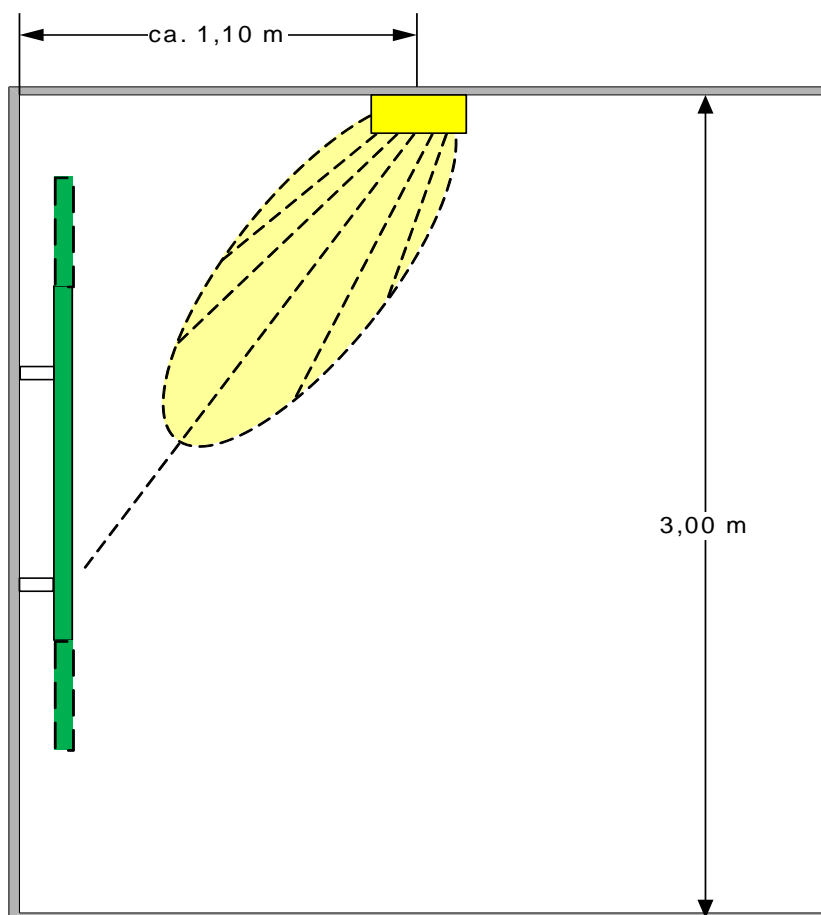
Abbildung 15: Separate Tafelbeleuchtung
