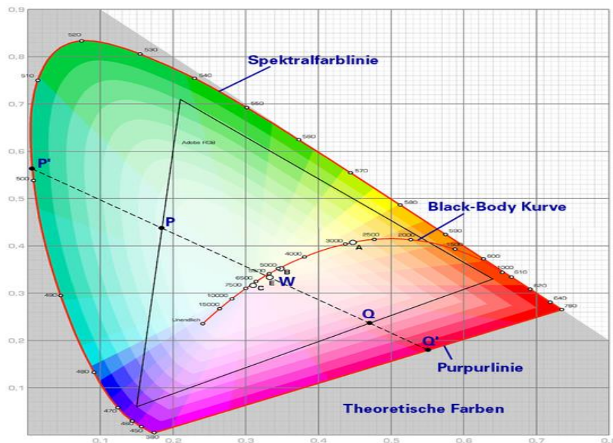
Abbildung 4: CIE-Normfarbtafel [62]
