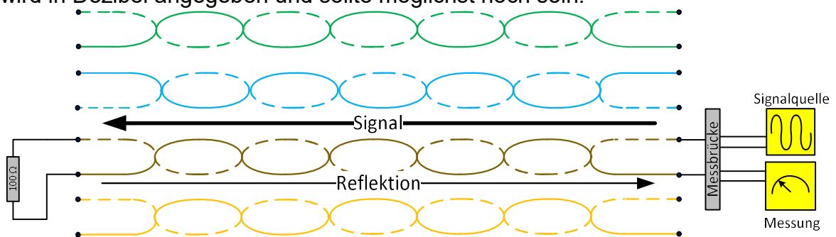
Abbildung 61: Rückflussdämpfung
