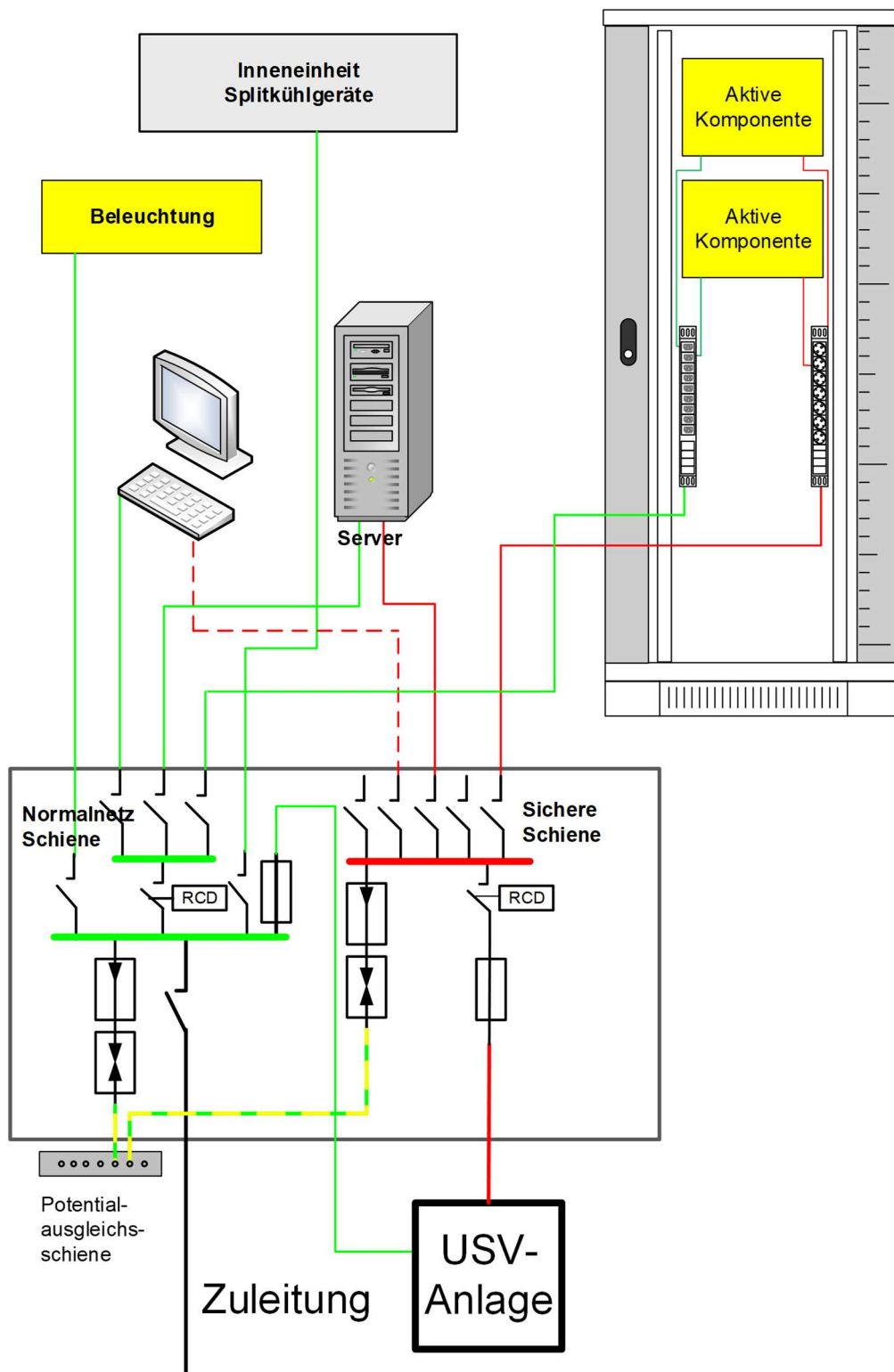
Abbildung 44: Stromversorgung Datenverteilerzimmern
