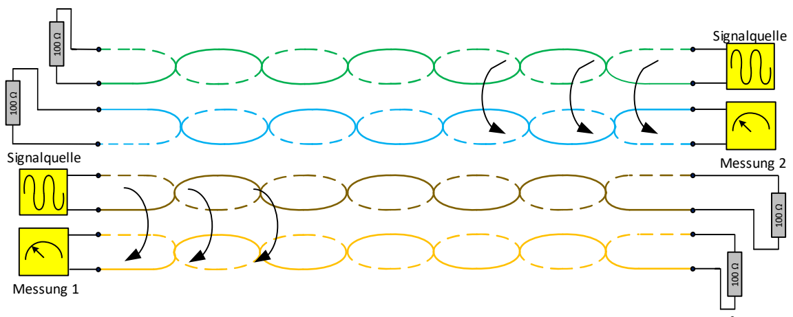
Abbildung 62: Nahnebensprehdämpfung
