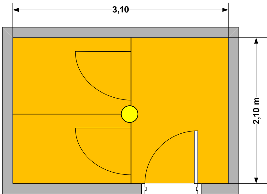
Abbildung 25: Sanitärraum1 LED-Leuchte 21,5 W / 2.600 lm (DIN EN 12464-1, Ref. Nr. 10.4)
