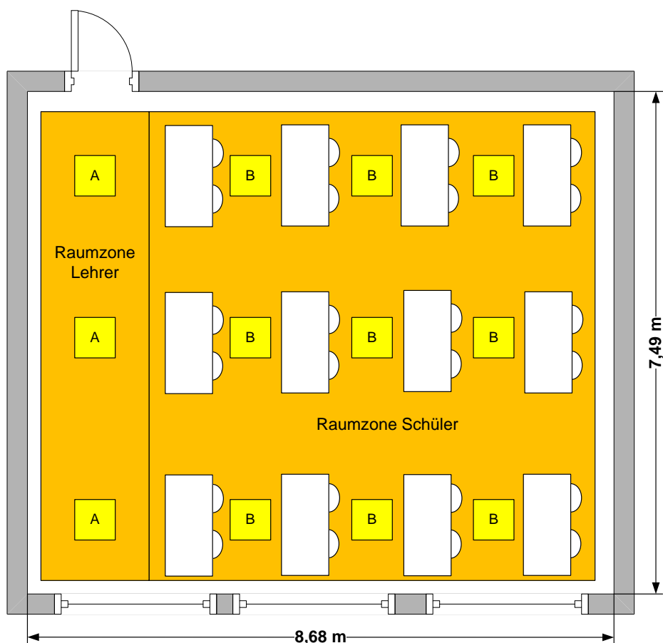
Abbildung 19: Beleuchtung eines Klassenzimmers (DIN EN 12464-1, Ref. Nr. 44.1)
