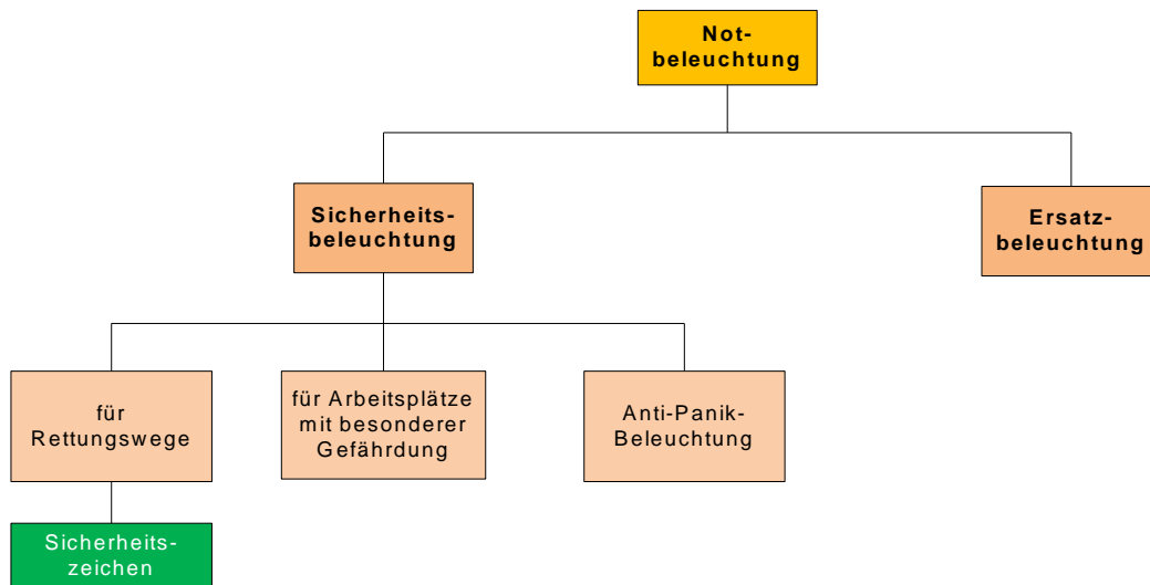
Abbildung 27: Systematik der Notbeleuchtung
