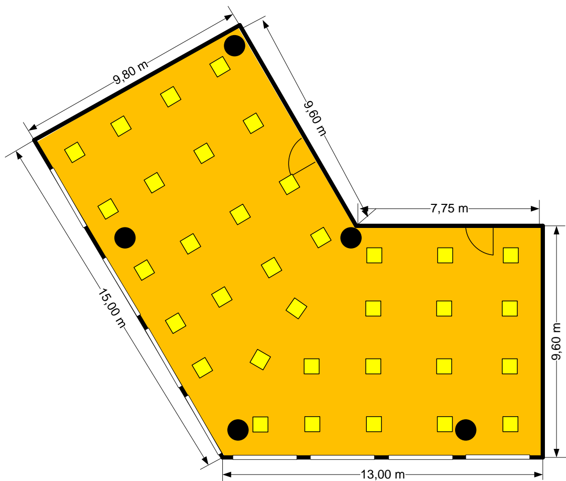
Abbildung 18: Großraumbüro (DIN EN 12464-1, Ref. Nr. 34.2)
