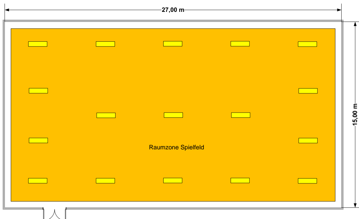
Abbildung 22: Beleuchtung einer Turnhalle 14 m x 26 m (DIN EN 12464-1, Ref. Nr. 44.26)
