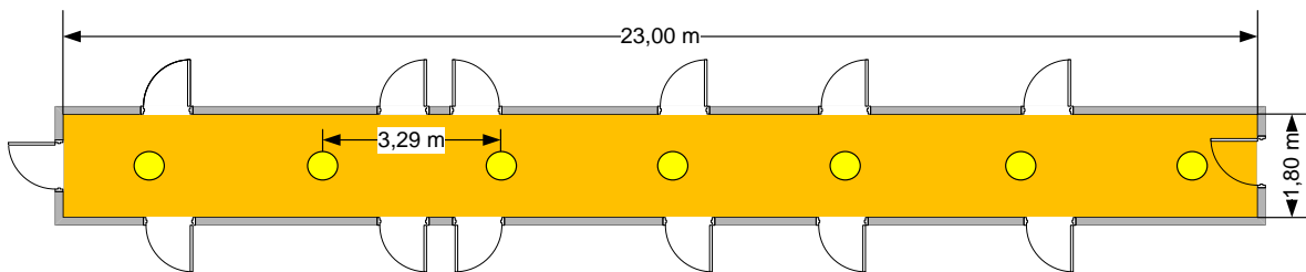
Abbildung 24: Flur (Einbauleuchten) (DIN EN 12464-1, Ref. Nr. 9.1)
