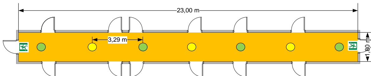
Abbildung 28: Flur mit Sicherheitsbeleuchtung (grün hinterlegt)
