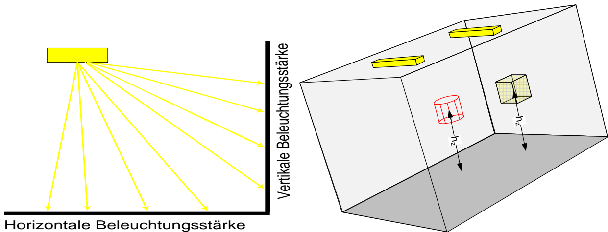
Abbildung 4: Schematische Darstellung von horizontaler bzw. vertikaler Beleuchtungsstärke (links) und zylindrischer Beleuchtungsstärke (rechts)
