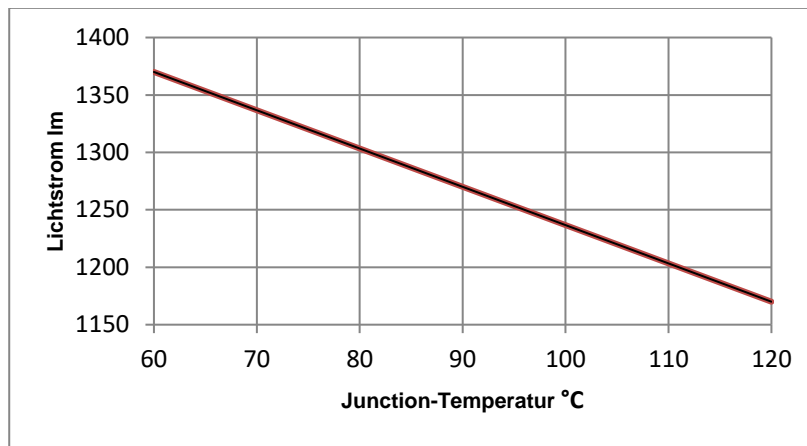
Abbildung 13: Beispielhafter Lichtstrom in Abhängigkeit von der Junction-Temperatur [72].
