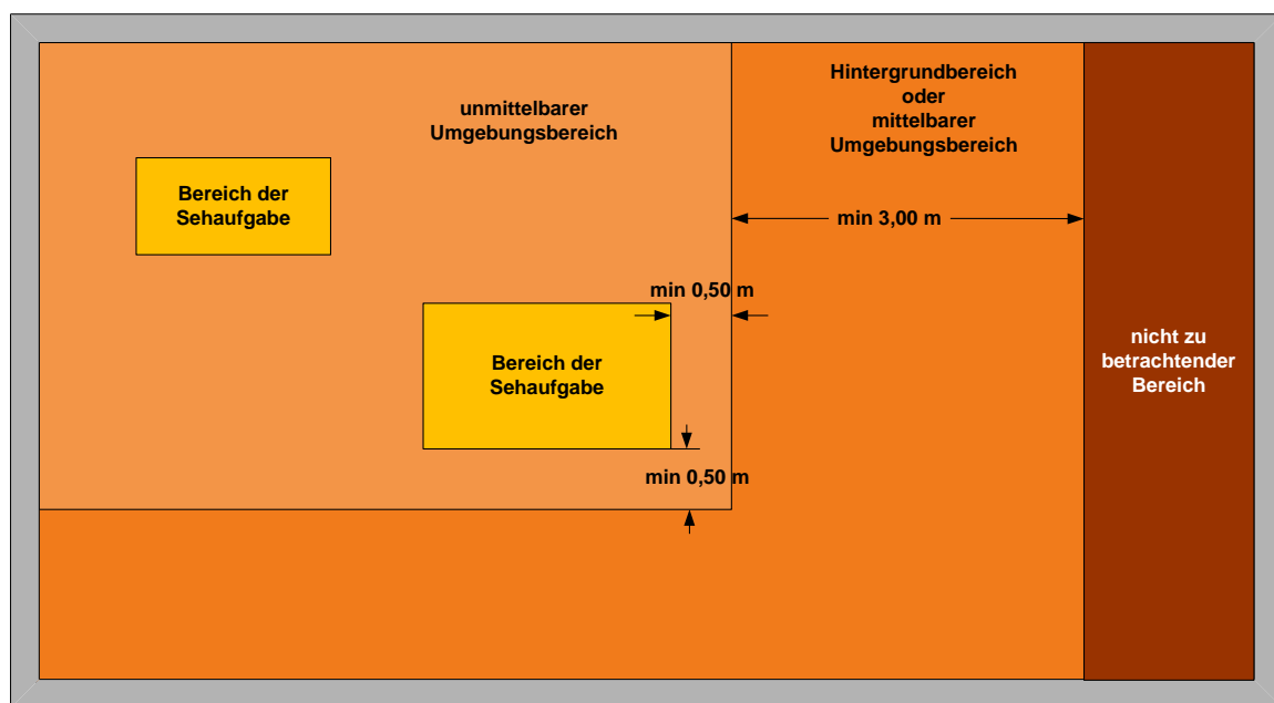
Abbildung 7: Ausbildung der lichttechnischen Bereiche nach DIN EN 12464-1
