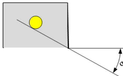
Abbildung 9: Abschirmwinkel \alpha bei Leuchten mit direkt sichtbarer Lichtquelle
