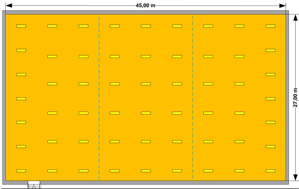
Abbildung 23: Beleuchtung einer Wettkampf-Sporthalle 27 m x 45 m
