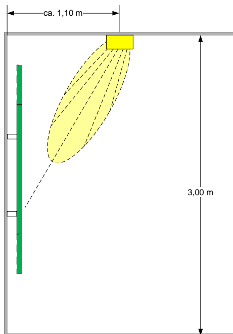
Abbildung 20: Separate Tafelbeleuchtung
