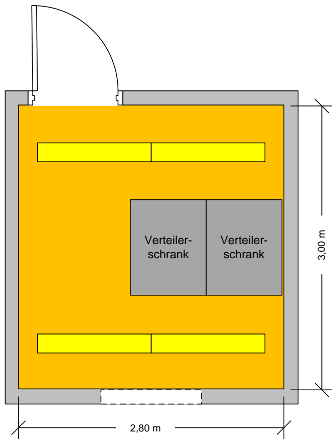
Abbildung 26: Datenverteilteraum
