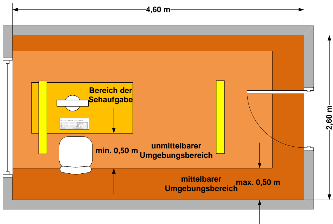
Abbildung 15: 1-Personen-Büro (DIN EN 12464-1, Ref. Nr. 34.2)
