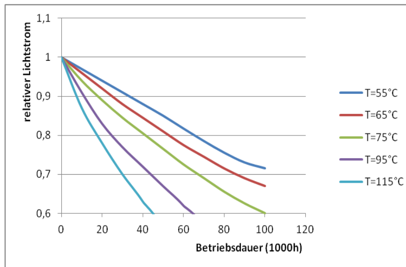
Abbildung 14: Beispielhafte relative Lichtströme in Abhängigkeit von der Junction-Temperatur und Betriebsdauer [72].
