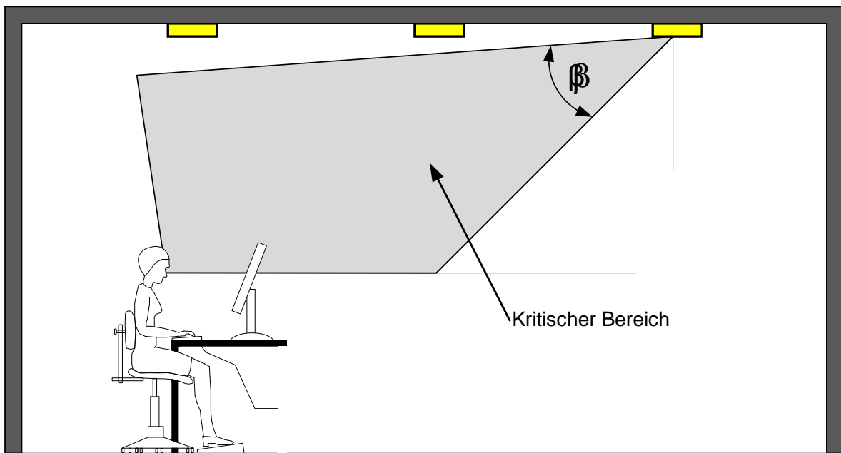
Abbildung 8: Kritischer Bereich für Direktblendung
