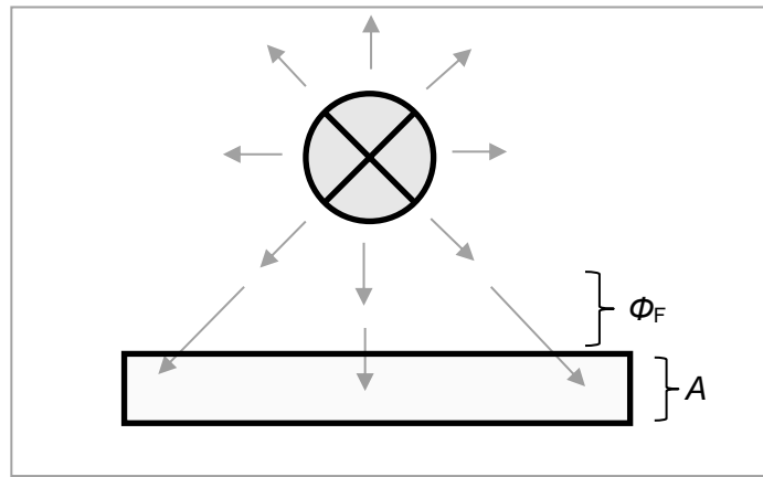
Abbildung 3: Schematische Darstellung der Beleuchtungsstärke E (Lichtstrom \Phi_F auf der Fläche A )
