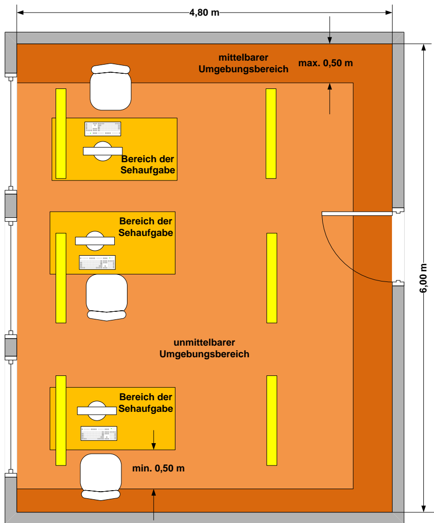
Abbildung 17: 3-Personen-Büro (DIN EN 12464-1, Ref. Nr. 34.2)
