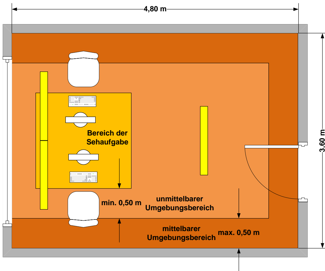
Abbildung 16: 2-Personen-Büro (DIN EN 12464-1, Ref. Nr. 34.2)
