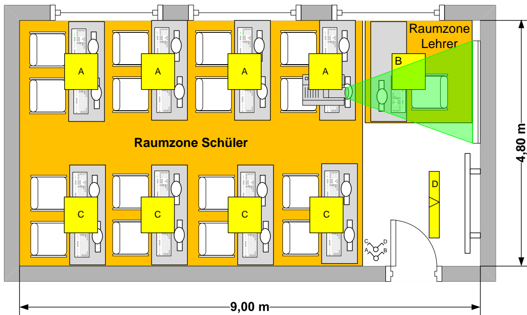
Abbildung 21: EDV-Schulungsraum (DIN EN 12464-1, Ref. Nr. 44.11)
