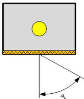
Abbildung 10: Ausstrahlungswinkel \gamma bei mittels durchleuchtenden optischen Elementen abgeschirmten Lichtquellen
