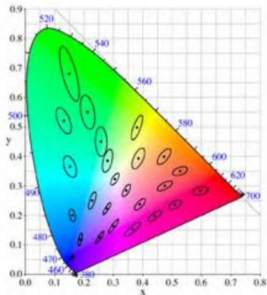
Abbildung 12: MacAdam-Ellipsen, zur Verdeutlichung 10-fach vergrößert.
