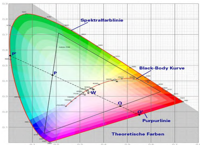
Abbildung 11: CIE-Normfarbtafel
