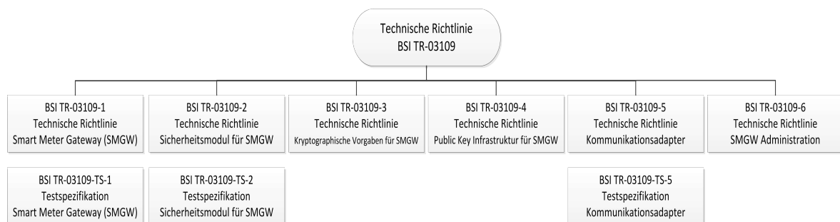
Abbildung 1: Dokumentenstruktur der BSI TR-03109
