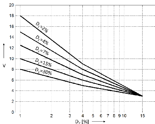
Bild 4-2: Ermittlung des Spektren-Überhöhungsfaktors
