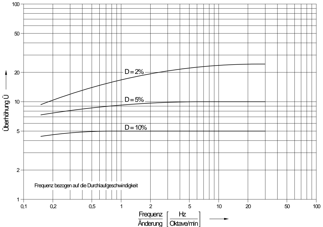
Bild 5-2: Überhöhungsfaktoren bei Gleitsinusanregung
