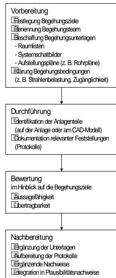
Bild 7-1: Ablaufschema Begehungen
