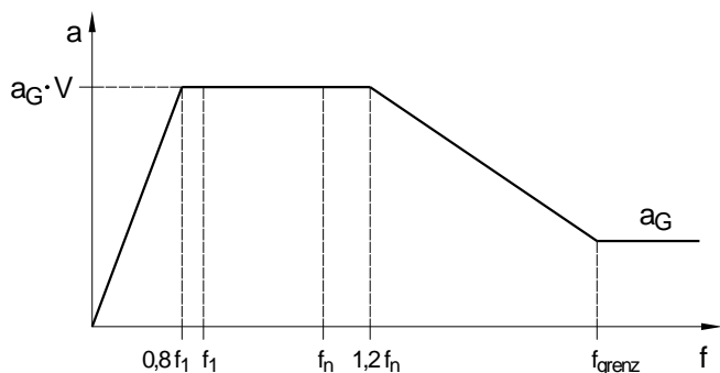
Bild 4-1: Ermittlung der Form des Antwortspektrums
