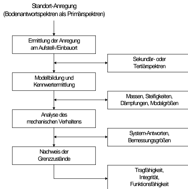
Bild 3-1: Übersicht über die Nachweisführung
