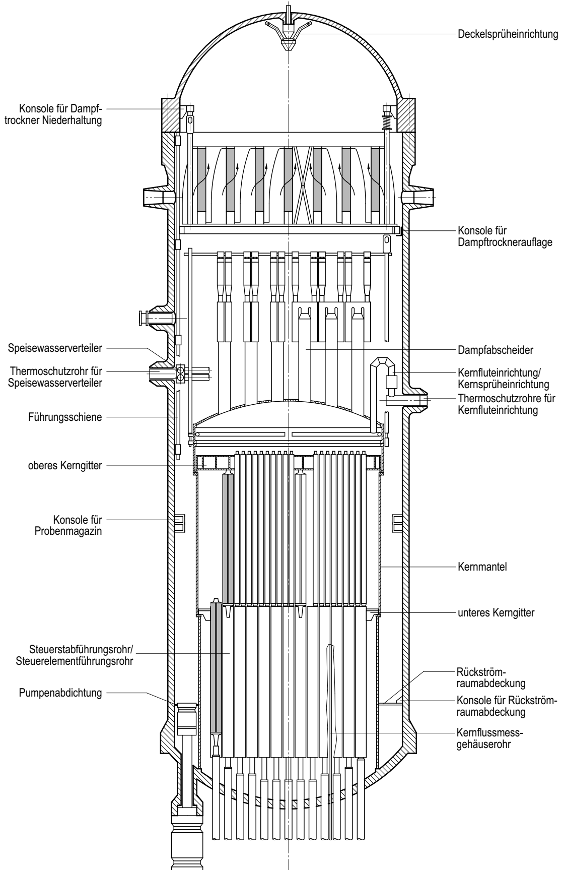
Bild 3-2: Darstellung typischer RDB-Einbauten (SWR)
