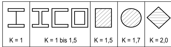
Bild C-1: Stützziffern (siehe Abschnitt C 2.2.1)
