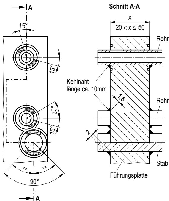
Bild 8-10: Abmessung des Prüfstücks für geschweißte Steuerstabführungseinsätze
