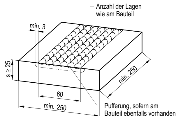
Bild 8-7: Abmessung des Prüfstücks für Hartauftragsschweißungen
