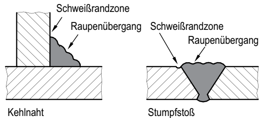
Bild 8-1: Erläuterung der Begriffe Kerbe, Schweißrandzone und Raupenübergang
