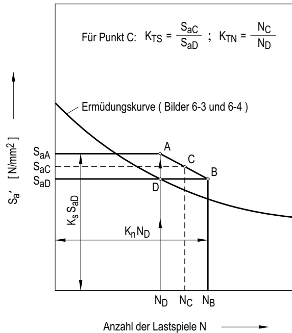
Bild D-2: Diagramm zur Ermittlung der Versuchsparameter (siehe Abschnitt D 3.3 (3))
