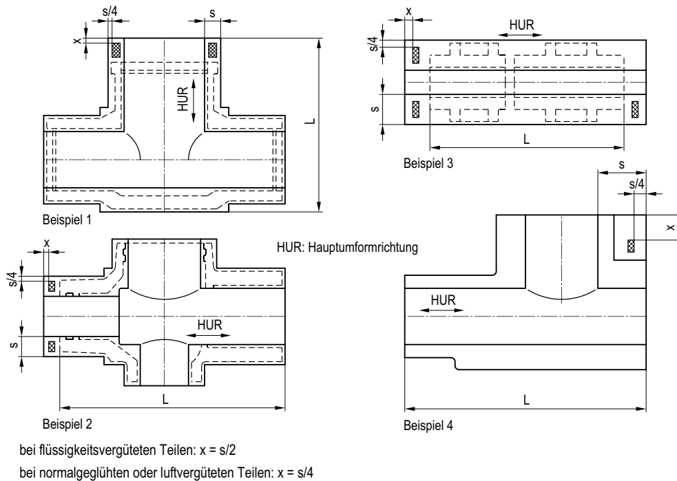
Bild 5.3-2: Beispiele für die Probenentnahme an geschmiedeten Armaturengehäusen
