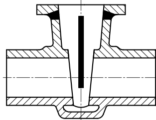
Keilschiebergehäuse
