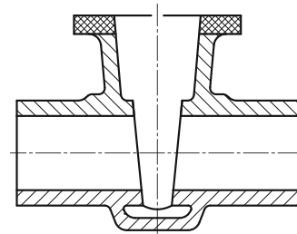
Bild 11.8-3: Keilschiebergehäuse
