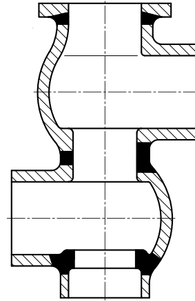
Mehrwegeventilgehäuse
