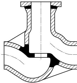
Durchgangsventilgehäuse
