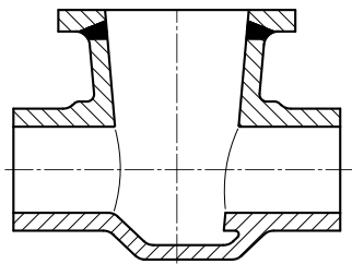
Rückschlagklappengehäuse
