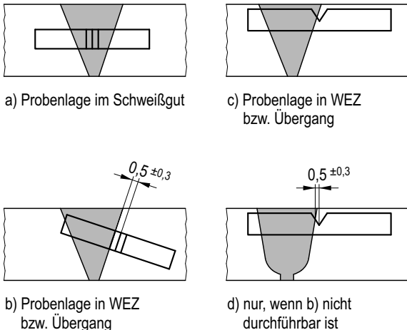
Bild B-1: Lage des Kerbs bei Kerbschlagbiegeproben
