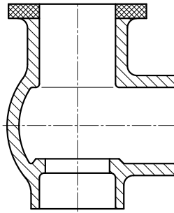
Bild 11.8-2: Eckventilgehäuse
