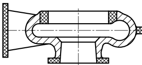
Bild 11.8-5: Mehrwegeventilgehäuse
