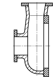
Bild 11.8-10: Ringgehäuse
