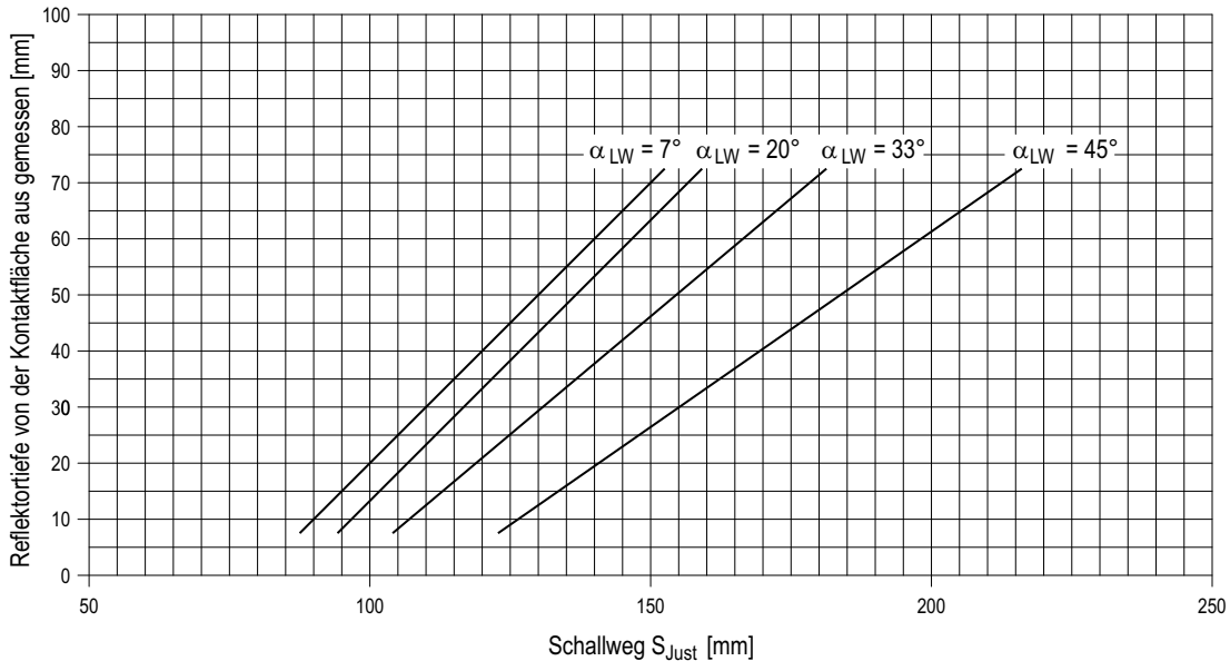
Bild D-19: Beispiel für LLT-Reflektortiefenmaßstäbe
