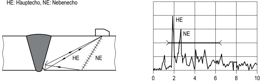
Bild D-16: Prüfung von Komponenten mit Nennwanddicken größer als 8 mm und gleich oder kleiner als 20 mm mittels Longitudinalwellen (Prüfkopf 70 Grad SEL)
