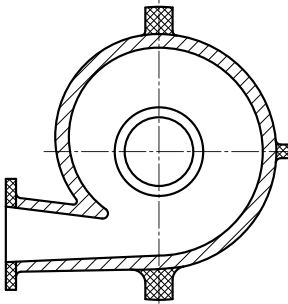
Bild 11.8-8: Spiralgehäuse
