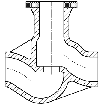
Bild 11.8-1: Durchgangsventilgehäuse
