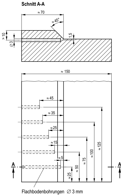
Bild D-10: Vergleichskörper für die Einstellung der Prüfempfindlichkeit bei Anwendung der Kriechwellentechnik (primäre Kriechwelle)
