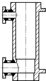
Topfpumpengehäuse
