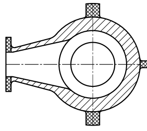
Bild 11.8-6: Druckgehäuse
