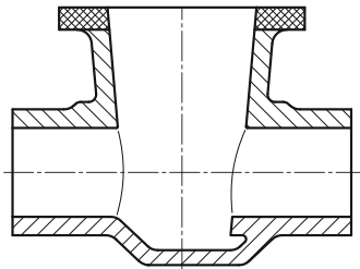
Bild 11.8-4: Rückschlagklappengehäuse
