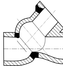
Schrägsitzventilgehäuse
