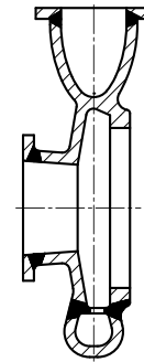
Doppelspiralgehäuse
