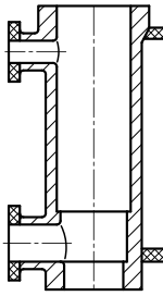
Bild 11.8-11: Topfpumpengehäuse
