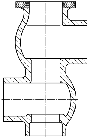
Bild 11.8-5: Mehrwegeventilgehäuse
