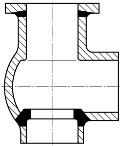
Eckventilgehäuse
