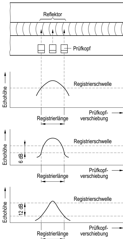
Bild D-20: Bestimmung der Registrierlänge
