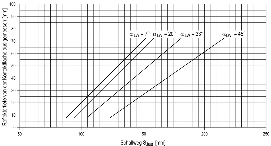
Bild D-19: Beispiel für LLT-Reflektortiefenmaßstäbe
