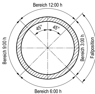
Skizze 1: Probenentnahmebereiche
