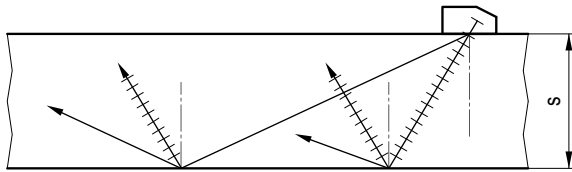
Bild D-13: Reflexion mit Wellenumwandlung beim Longitudinalwellen-Winkelprüfkopf
