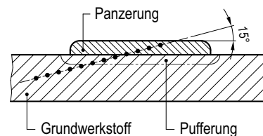
Bild 8-13: Härteprofil bei Panzerungen
