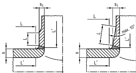
Bild 11-2: Beispiele für die konstruktive Gestaltung von Wanddickenübergängen unter Berücksichtigung der erforderlichen Prüflängen für die Ultraschallprüfung blechen bearbeiteter Stumpfnähte \geq DN 80 und s \geq 8 mm (gegenseitige Einschallung eingeschränkt)
