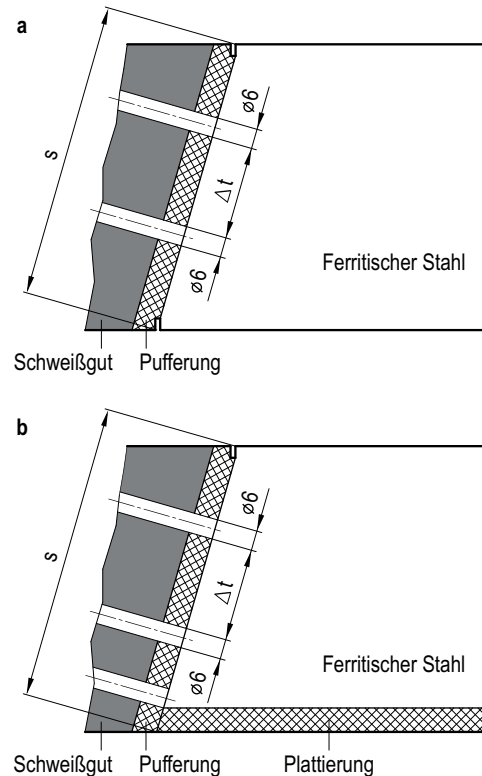
Bild 11-10: Lage der Flachbodenbohrungen und der Nuten für die Prüfung der Grenzfläche zum ferritischem Grundwerkstoff auf Bindung
