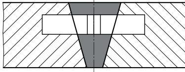
Skizze 2: Lage der Kerbschlagprobe in der Wärmeinflusszone
