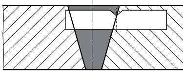
Skizze 4: Kerbschlagprobe gemäß DIN EN ISO 15614-1 in der Wärmeinflusszone
