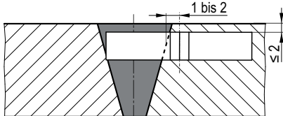
Skizze 4: Kerbschlagprobe gemäß DIN EN ISO 15614-1 in der Wärmeinflusszone
