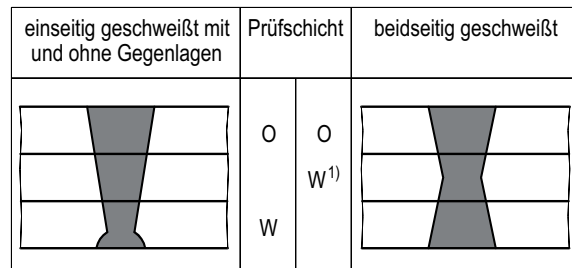
Bild 8-2: Prüfschichten bei ferritischen Werkstoffen für s > 50 mm
