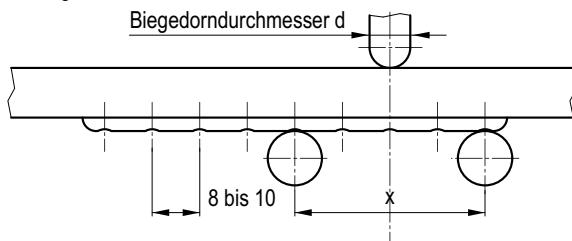
Bild 8-15: Risseinleitung in die Hartpanzerung
