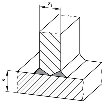
Bild 8-1: Wanddicken s und s_1 bei DHV-Schweißverbindung
