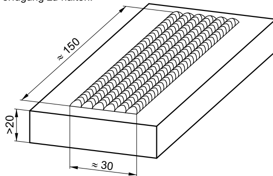
Bild 3-1: Prüfstück für das Schweißen von Panzerungen
