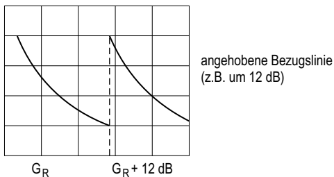
Bild D-4: Gestufte Bezugslinie
