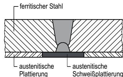
Bild 5-2: Verbindungsschweißung plattierter Bauteile
