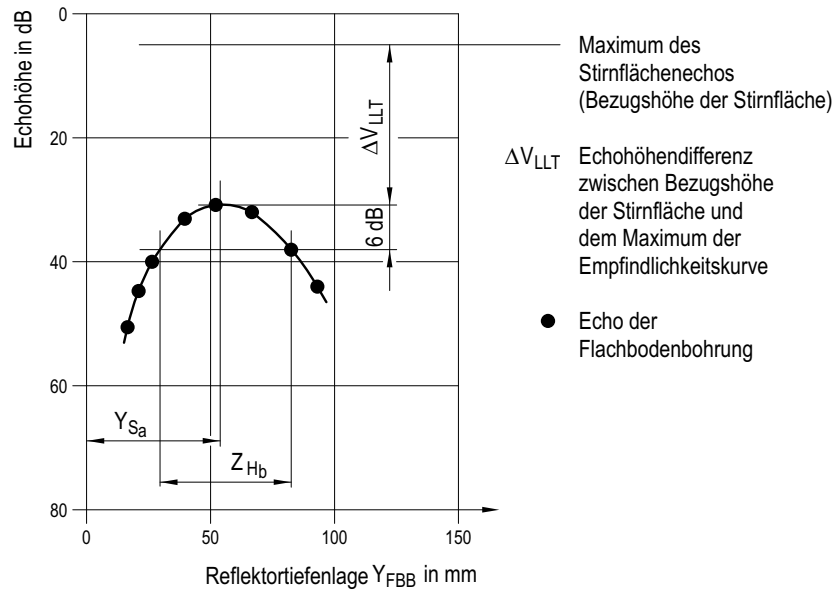
Bild D-18: Beispiel für ein LLT-Empfindlichkeitsdiagramm
