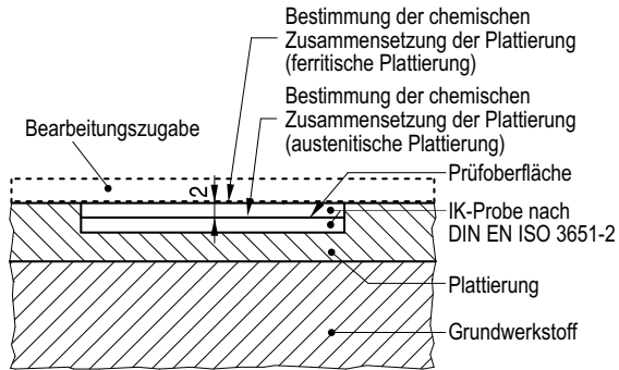
Skizze 1: Korrosionsprüfung und Prüfung der chemischen Zusammensetzung
