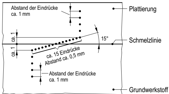
Skizze 2: Härteprüfung
