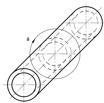
Skizze 3: Rohrposition für Schweißposition PK (Orbitalschweißen) a : Der Pfeil zeigt die Schweißfortschrittsrichtung
