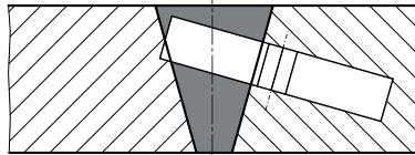
Skizze 2: Lage der Kerbschlagprobe in der Wärmeinflusszone
