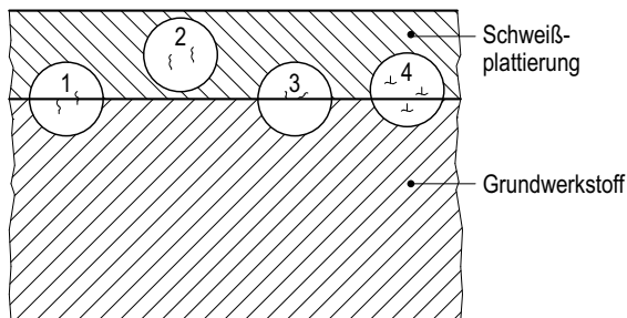
Bild 8-10: Probenlagen und Prüforte an Prüfstücken mit Auftragschweißungen
