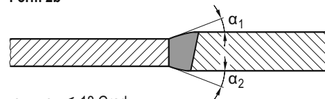
Bild 11-5: Beispiele für die prüfgerechte Gestaltung von Rund- und Längsnähten für die Durchstrahlungsprüfung
