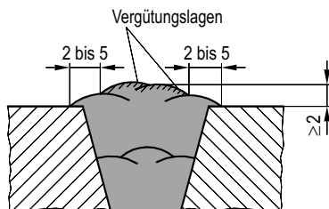
Bild 5-1: Vergütungslagentechnik ferritischer Schweißnähte am Beispiel der Schweißposition Wannenlage (PA)
