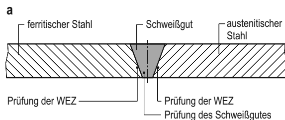
Bild 8-6: Lage der Härtereihe bei der Härteprüfung HV 5 an Querschleifen von ferritischen Verbindungsschweißungen
