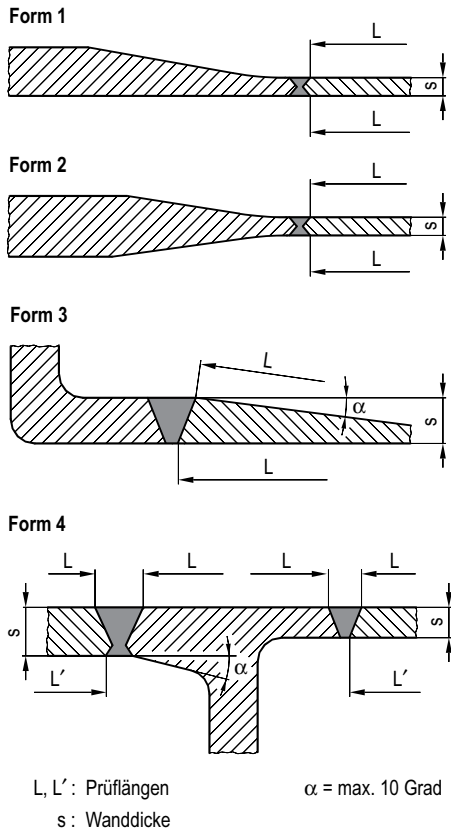
Bild 11-2: Beispiele für die konstruktive Gestaltung von Wanddickenübergängen unter Berücksichtigung der erforderlichen Prüflängen für die Ultraschallprüfung blechen bearbeiteter Stumpfnähte \geq DN 80 und s \geq 8 mm (gegenseitige Einschallung eingeschränkt)
