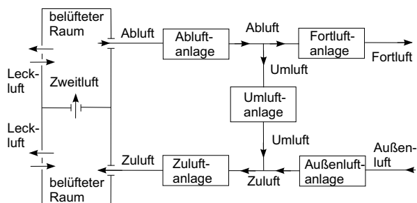
Bild 2-1: Benennungen von Luftströmen und Anlagen
