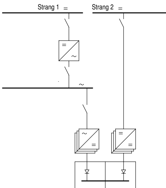
Bild 4-3: Beispiel eines Konzeptes mit redundanten Schaltnetzteilkombinationen zur Versorgung von leitentechnischen Einrichtungen
